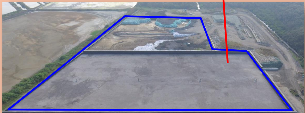
三期飛灰穩定化物掩埋空間尚餘13萬 m 3
