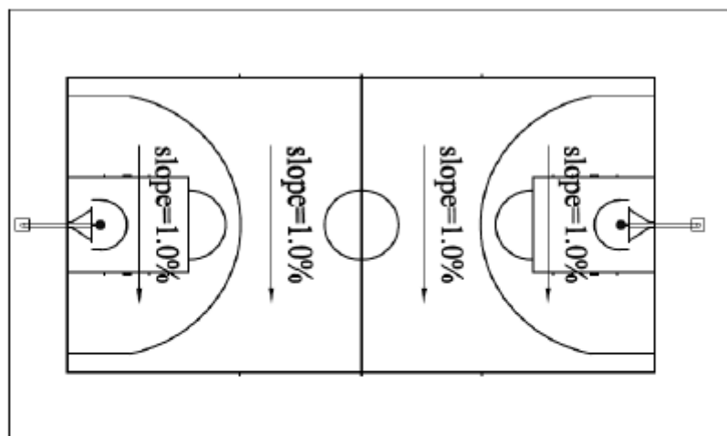
籃球場洩水坡度示意圖
