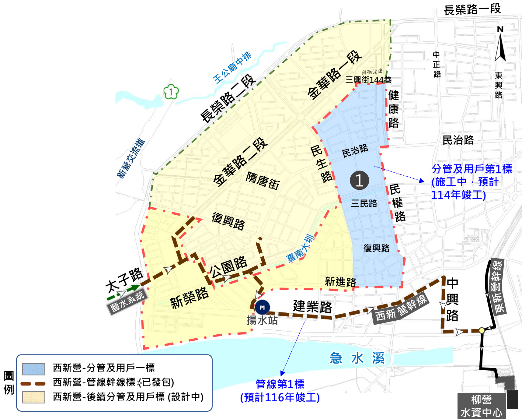
臺南市柳營污水下水道系統西新營分區工程範圍圖
