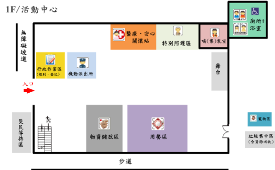
臺南市 中西區光賢里活動中心 避難收容處所平面配置圖
