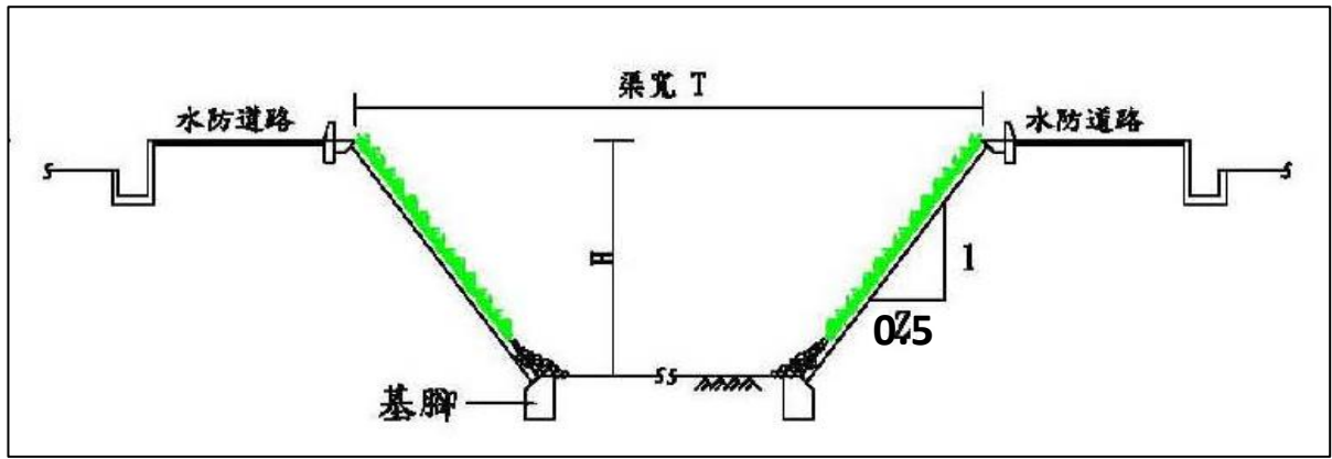
圖 2 排水設置示意圖
