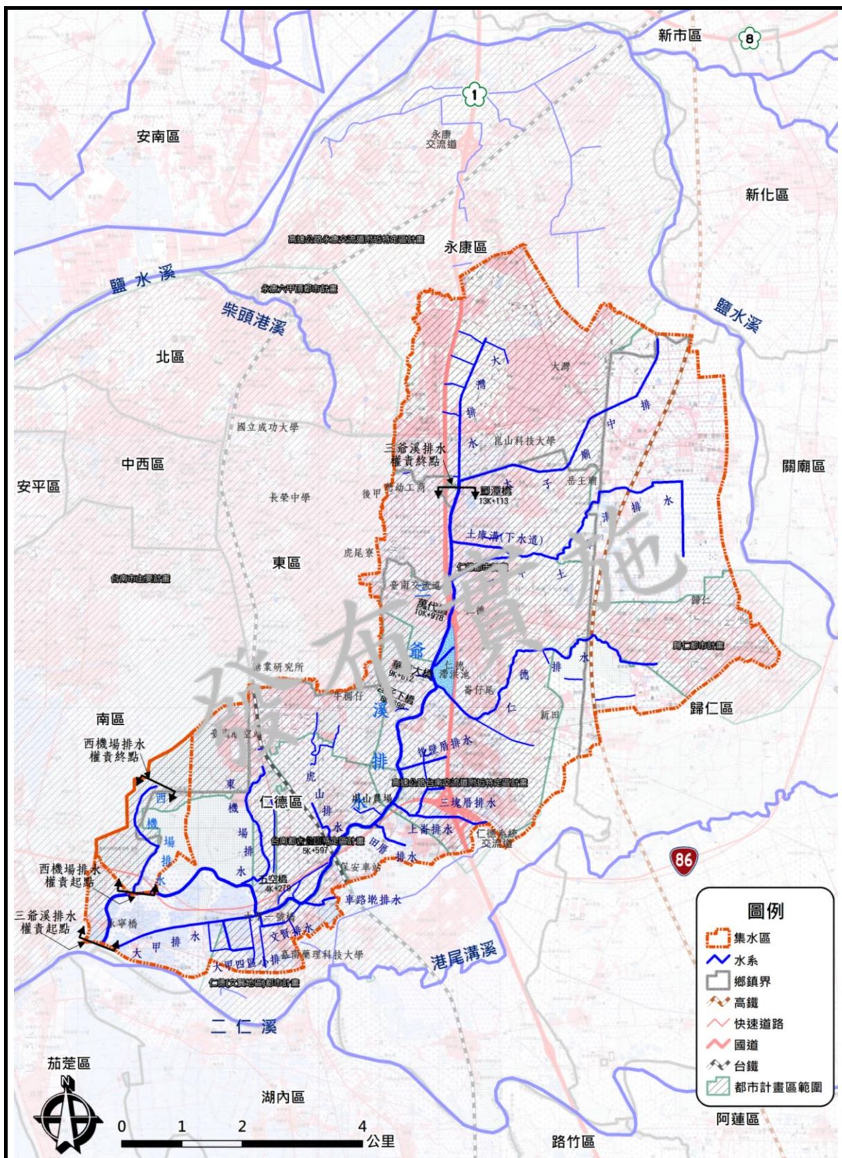
圖 6：三爺溪排水集水區範圍示意圖
