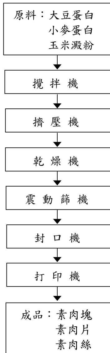
圖四 原廠區生產製造流程示意圖
