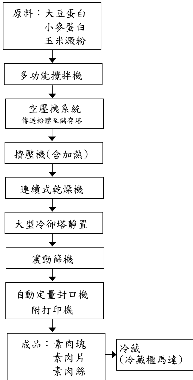
圖七 擴建後生產製造流程示意圖
