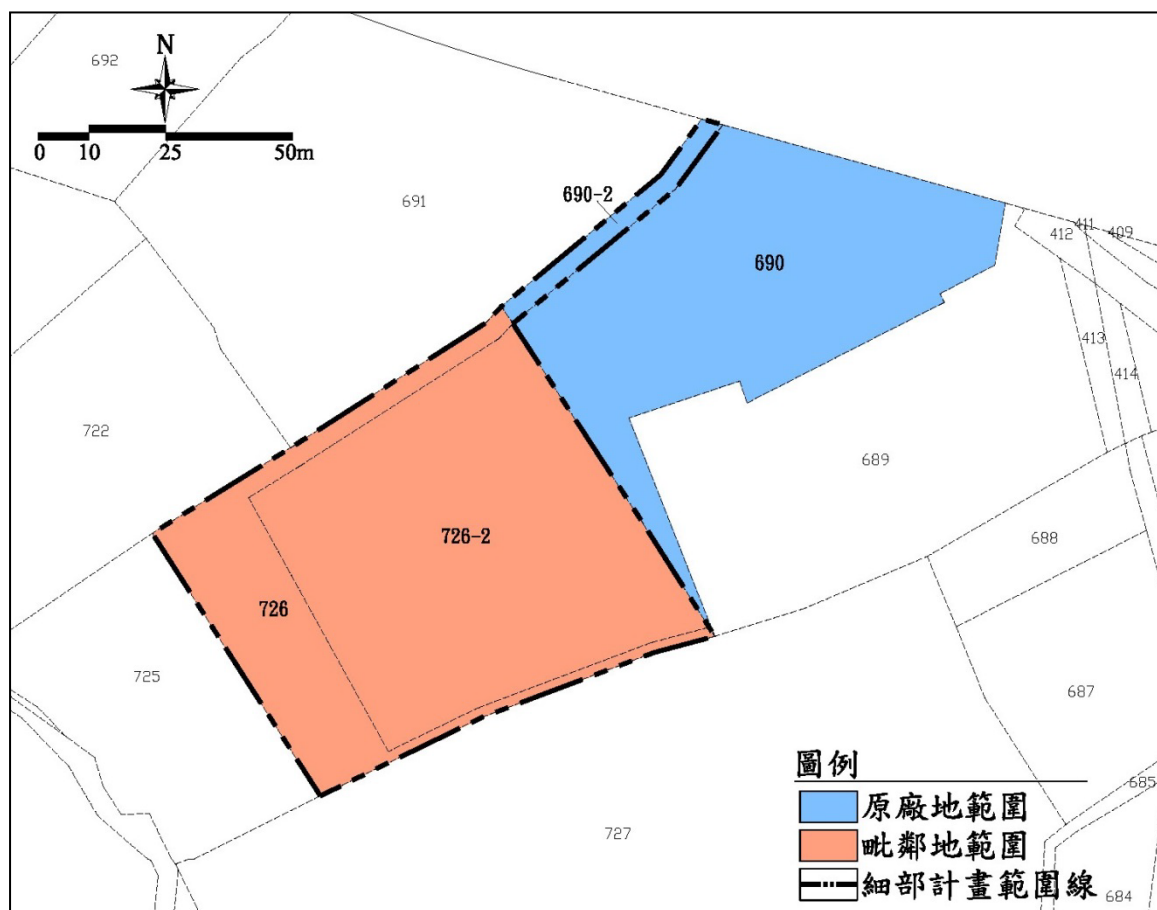
圖二 原廠地、毗鄰地暨細部計畫範圍地籍示意圖
