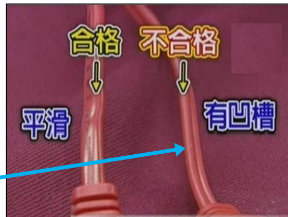
(b) 電源線雙層與單層的區別
