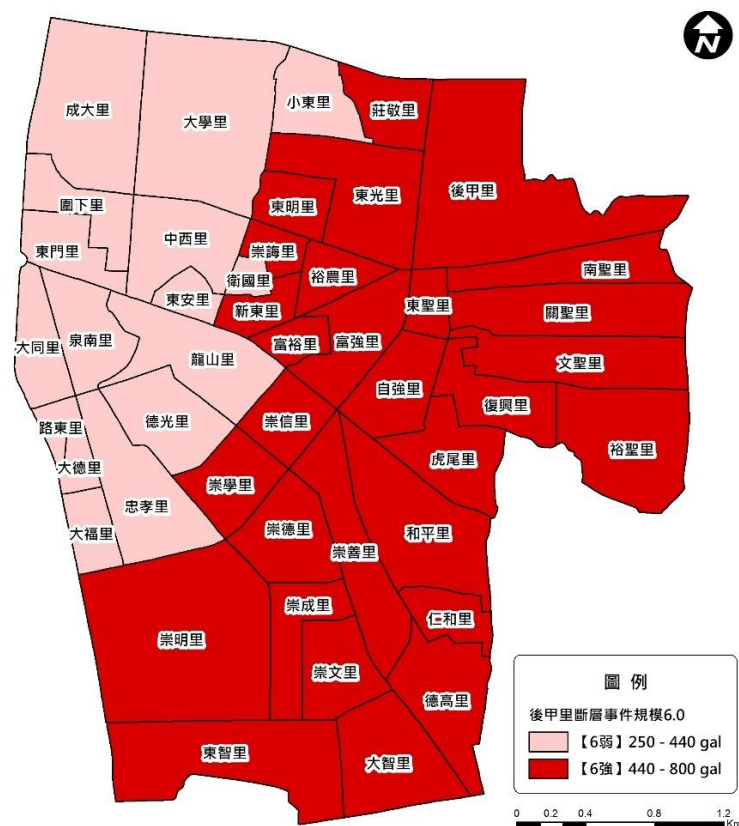
圖2、後甲里斷層事件東區各里最大地表加速度分布圖
