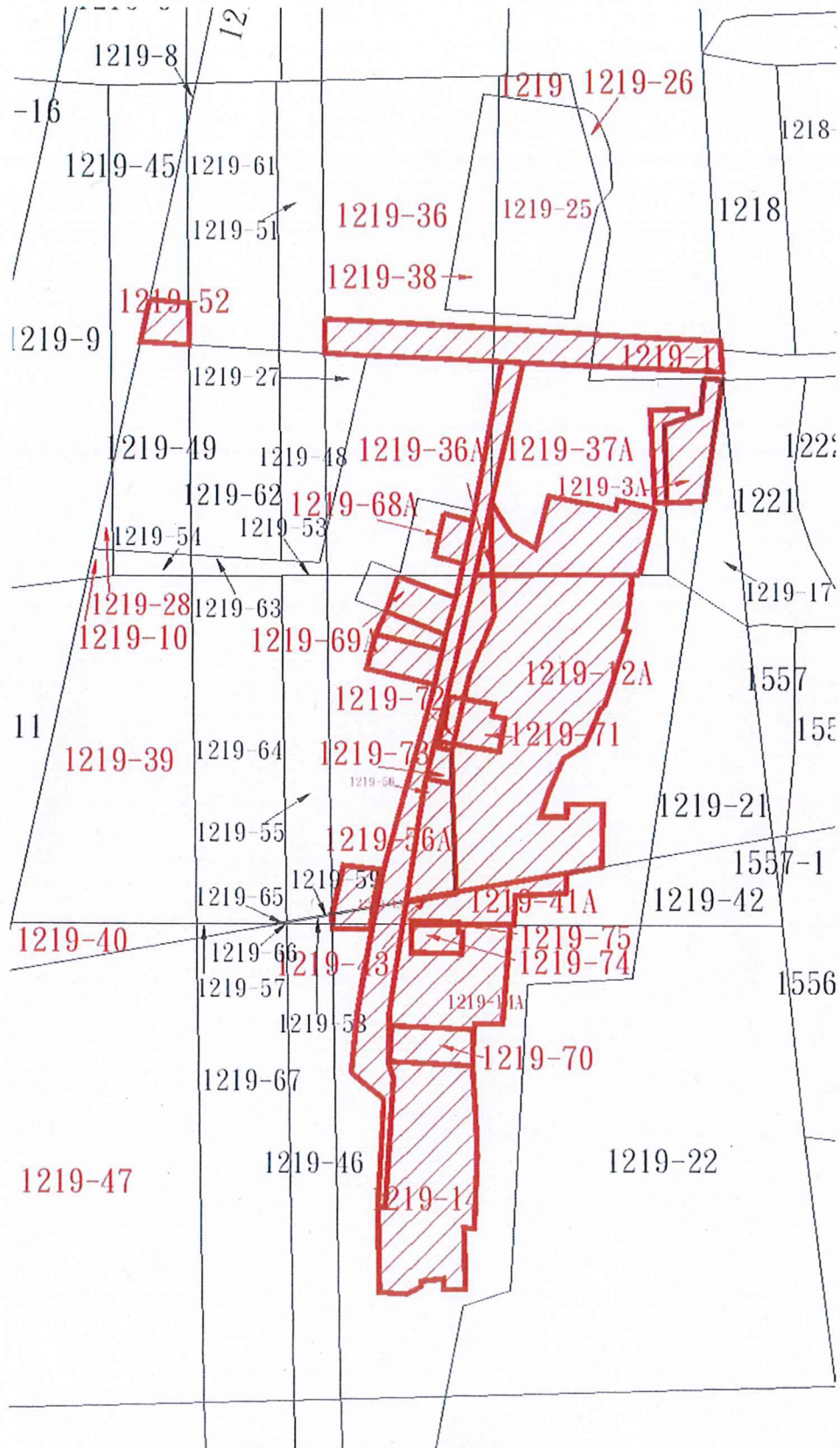
第 2102 號飛砂防止保安林解除圖三-不含正射影像(南區中和段)
