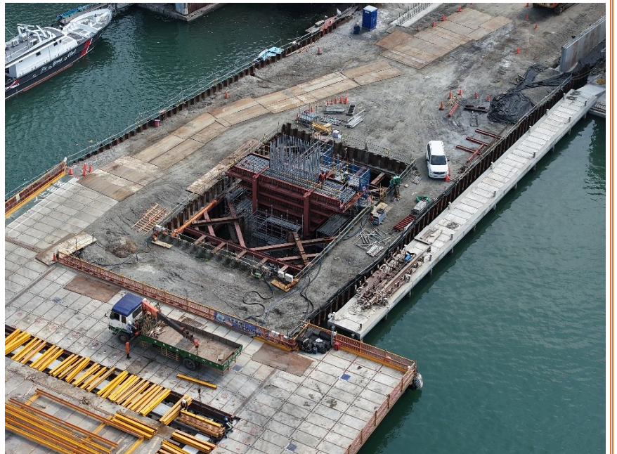
P7 橋墩帽梁施作
