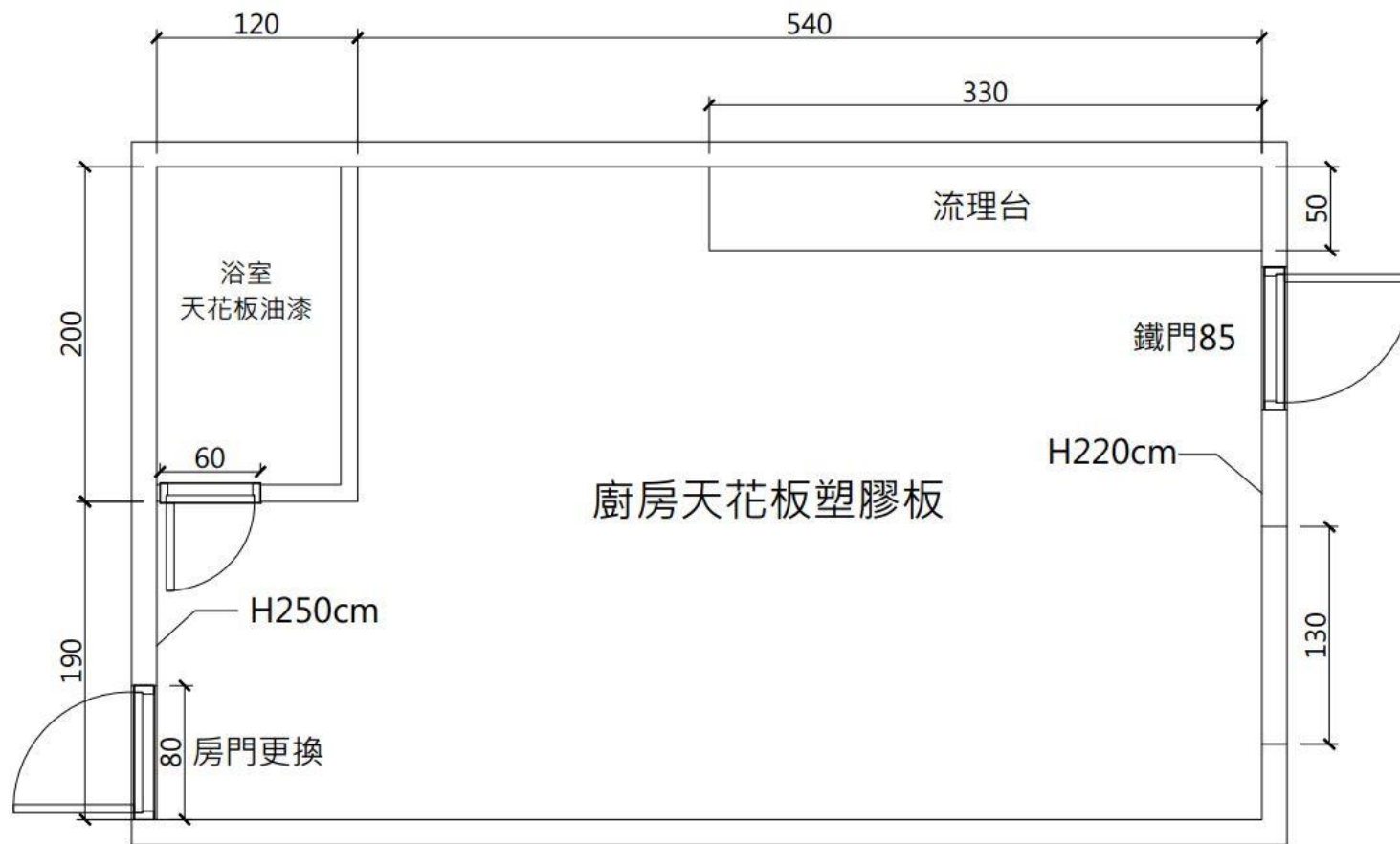
安定區安定里96-8號平面圖 A3=1:30
