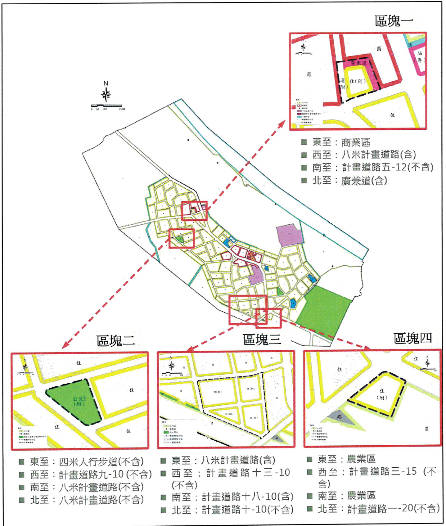
圖1-1：重劃區位置示意圖
