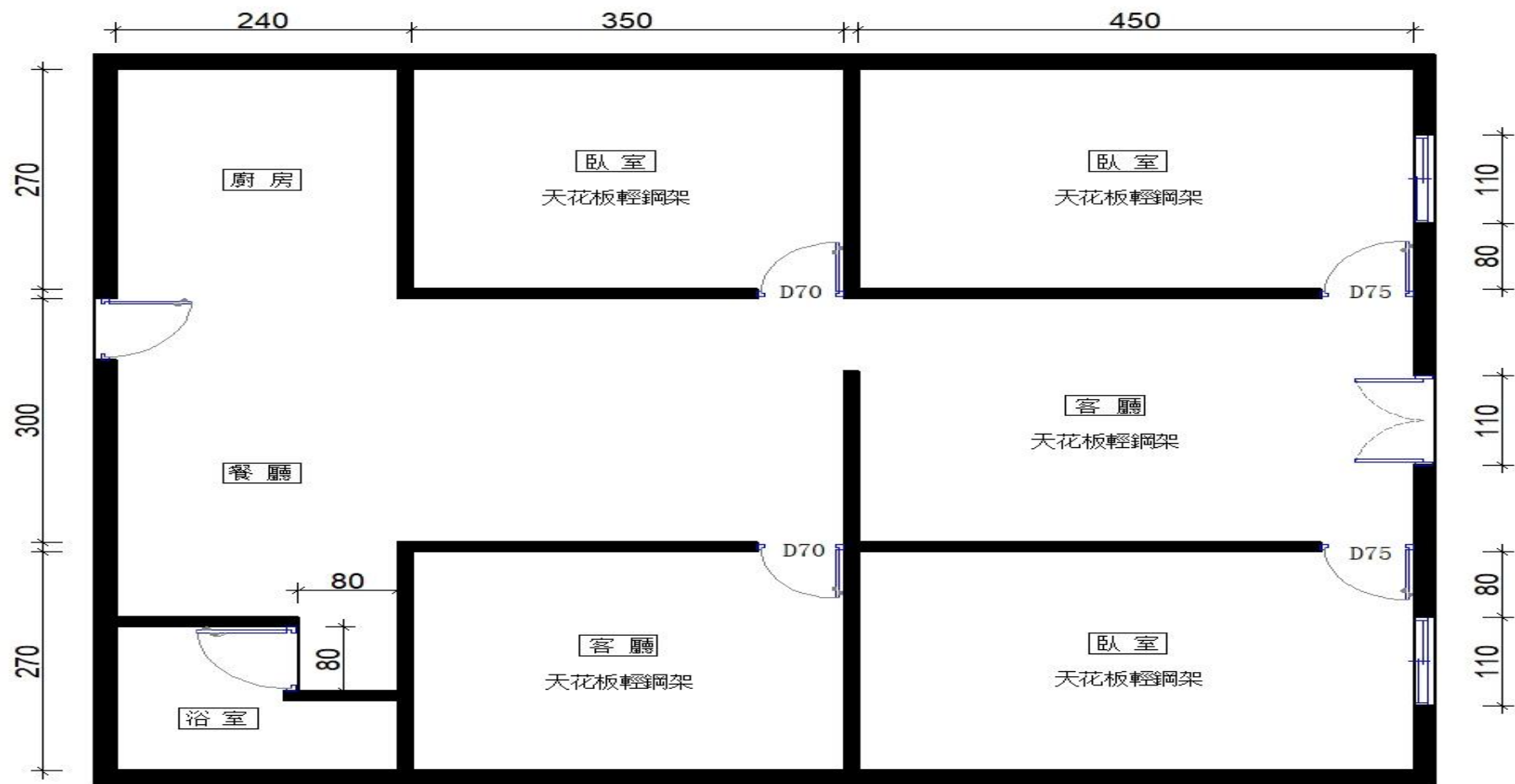
台南市麻豆區麻口里60號 平面圖
