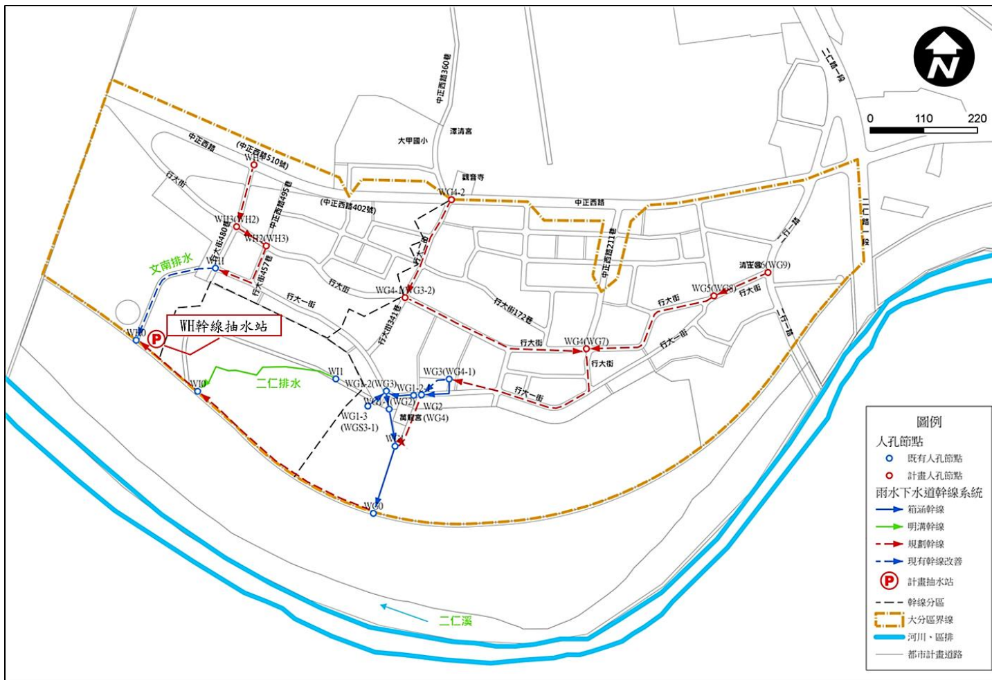
圖6 二仁排水分區雨水下水道系統改善平面圖
