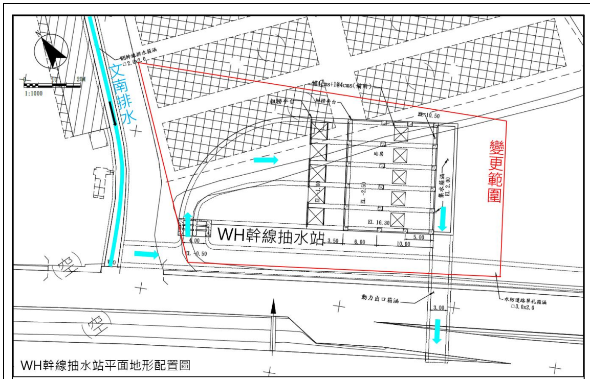
圖7 WH幹線抽水站平面地形配置圖
