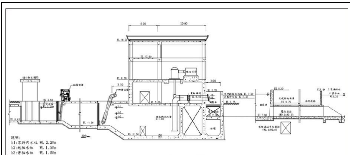
圖8 WH幹線抽水站縱剖面圖
