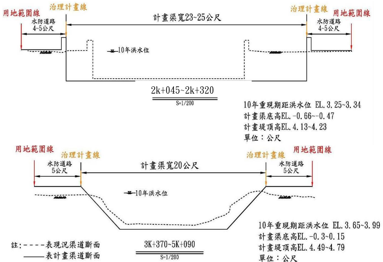
六塊寮排水橫斷面規劃示意圖
