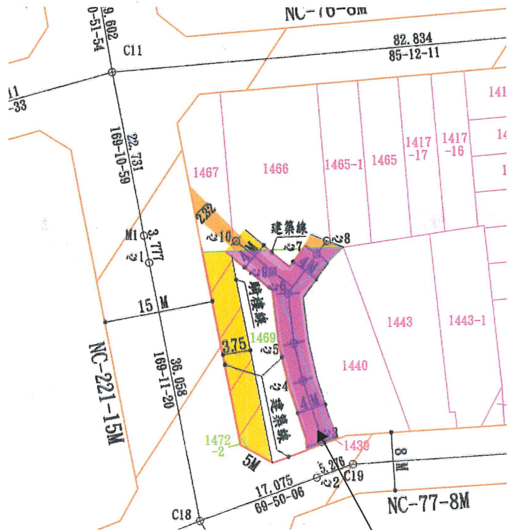
地籍套繪圖 S=1:500
