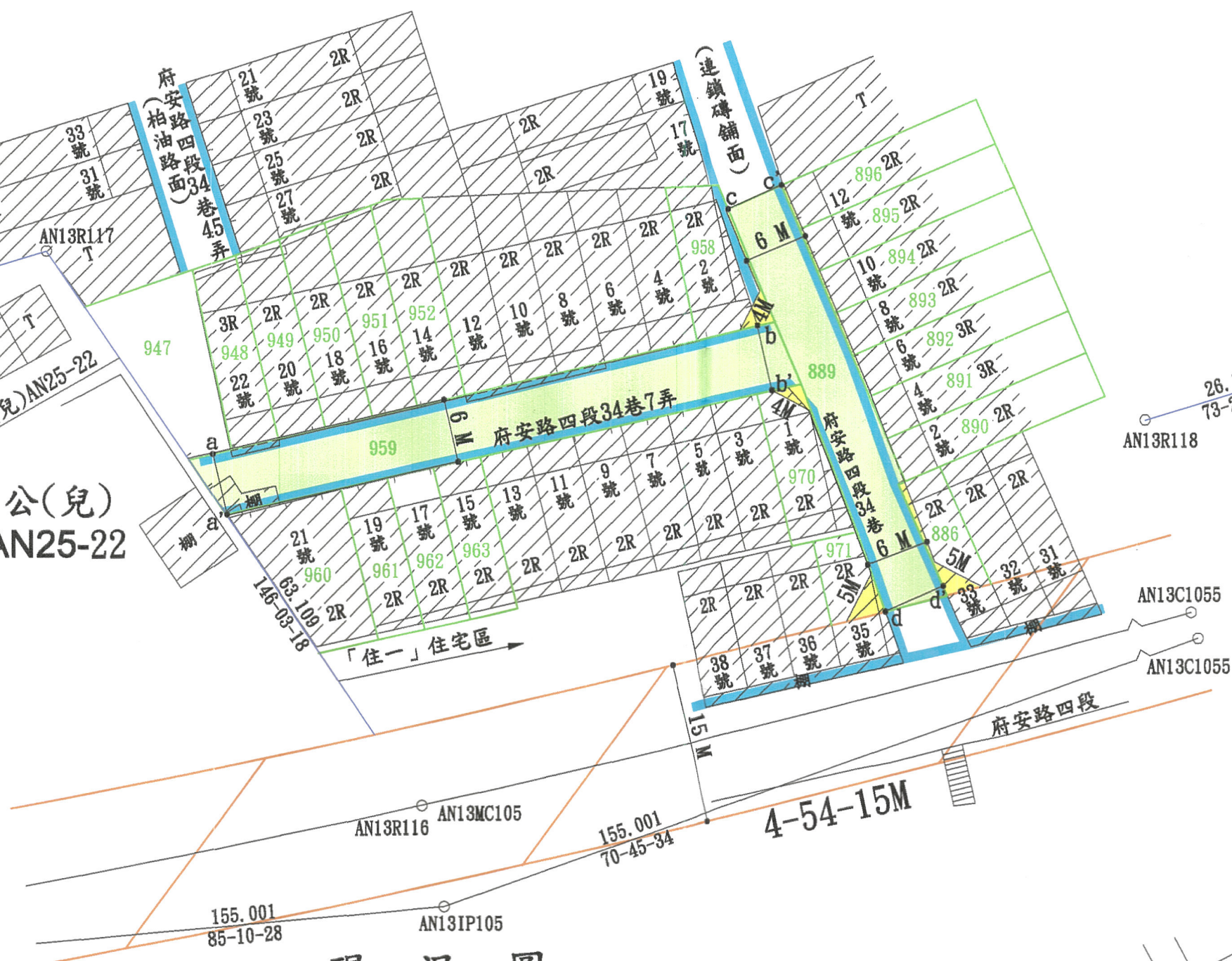
現況圖 比例尺:1/500
