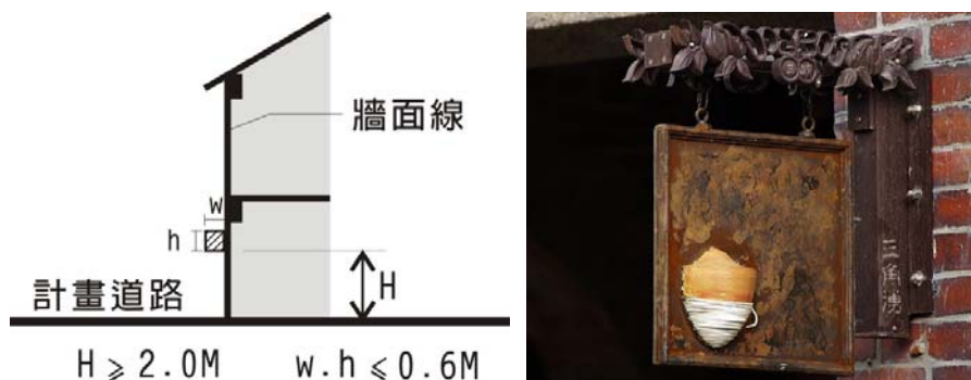
圖十八 側懸式招牌廣告設置說明圖
