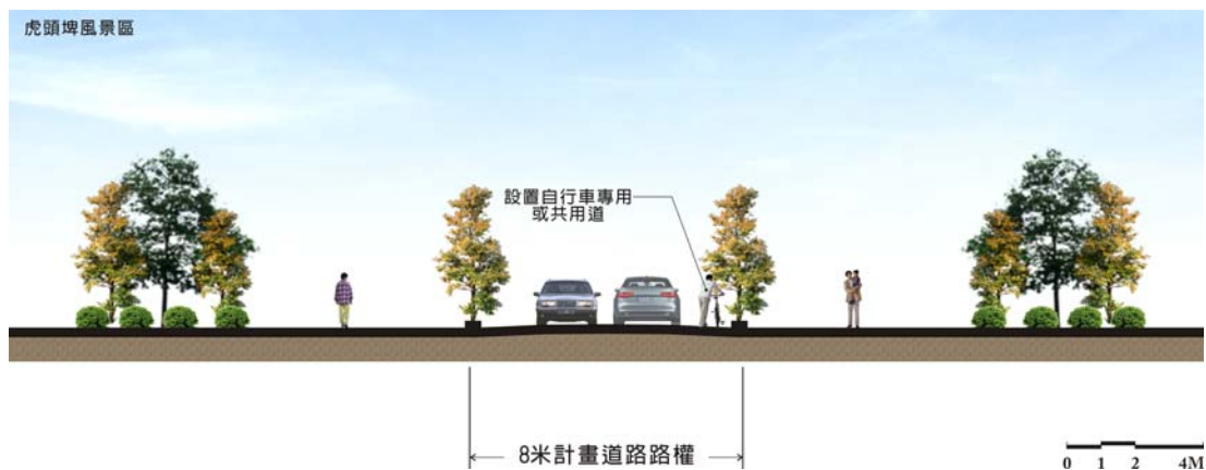
圖七 8 米計畫道路斷面示意圖
