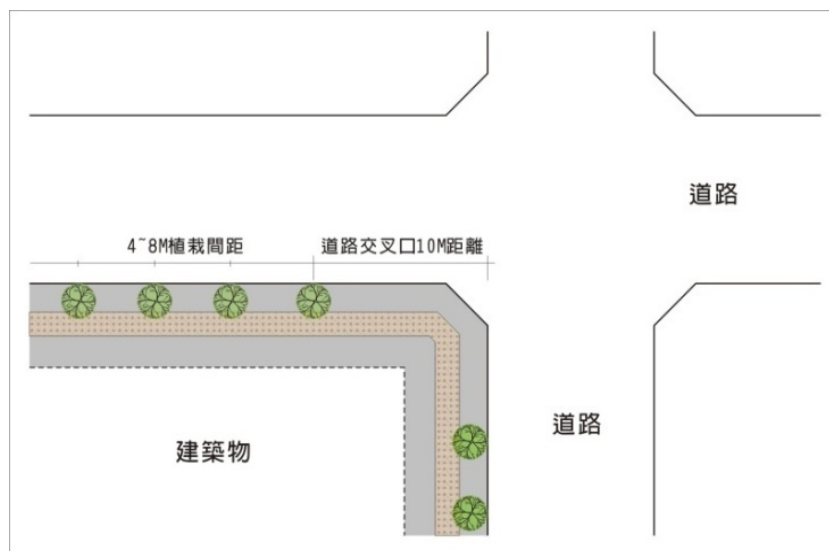
圖十二 行道樹植栽設置說明圖
