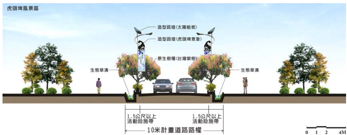
圖六 10 米計畫道路斷面示意圖
