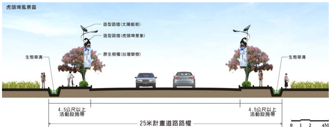
圖三 25 米計畫道路斷面示意圖
