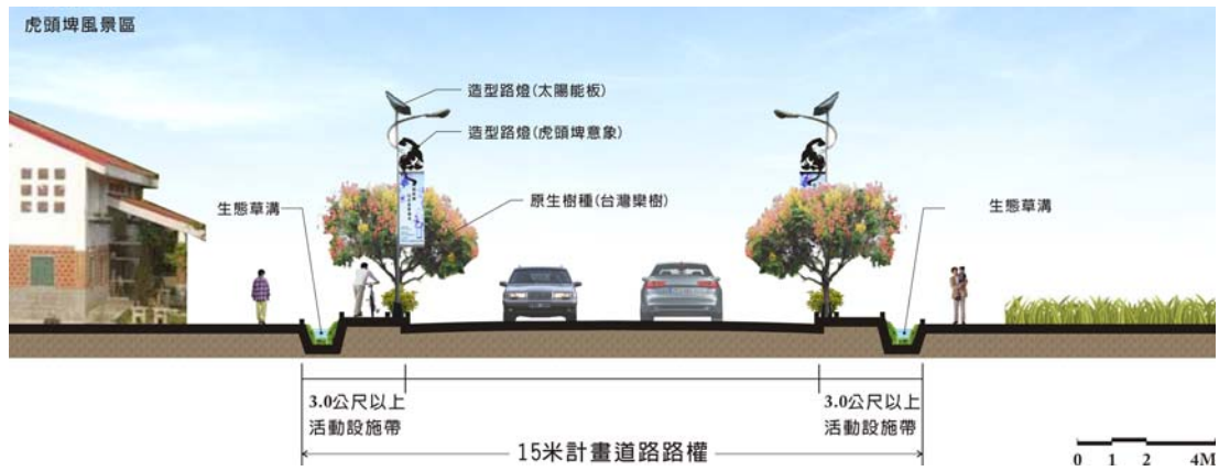
圖四 15 米計畫道路斷面示意圖
