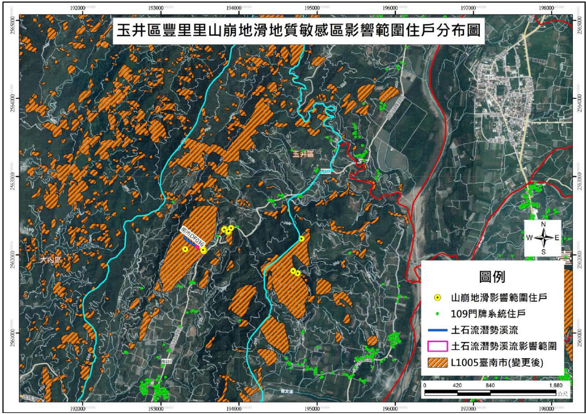
圖 4-1-6 豐里里山崩地滑地質敏感區影響範圍住戶分布圖
