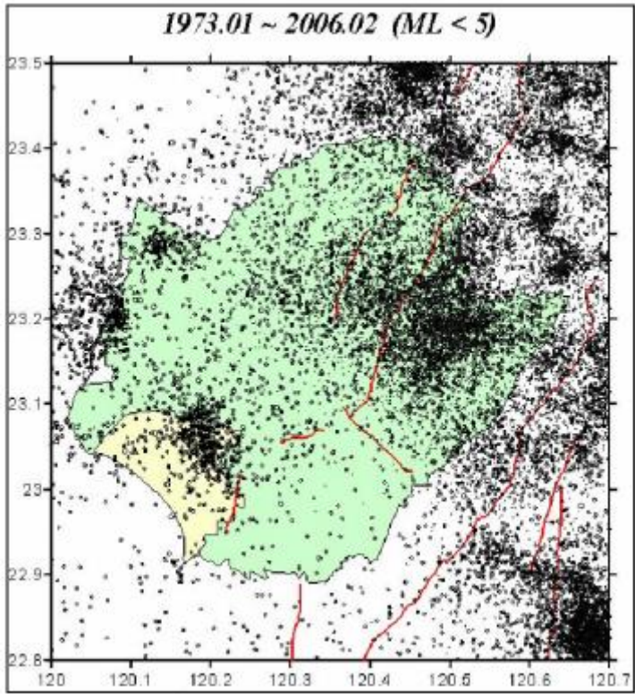
圖 6-2-2 臺南地區的地震活動與斷層分布
