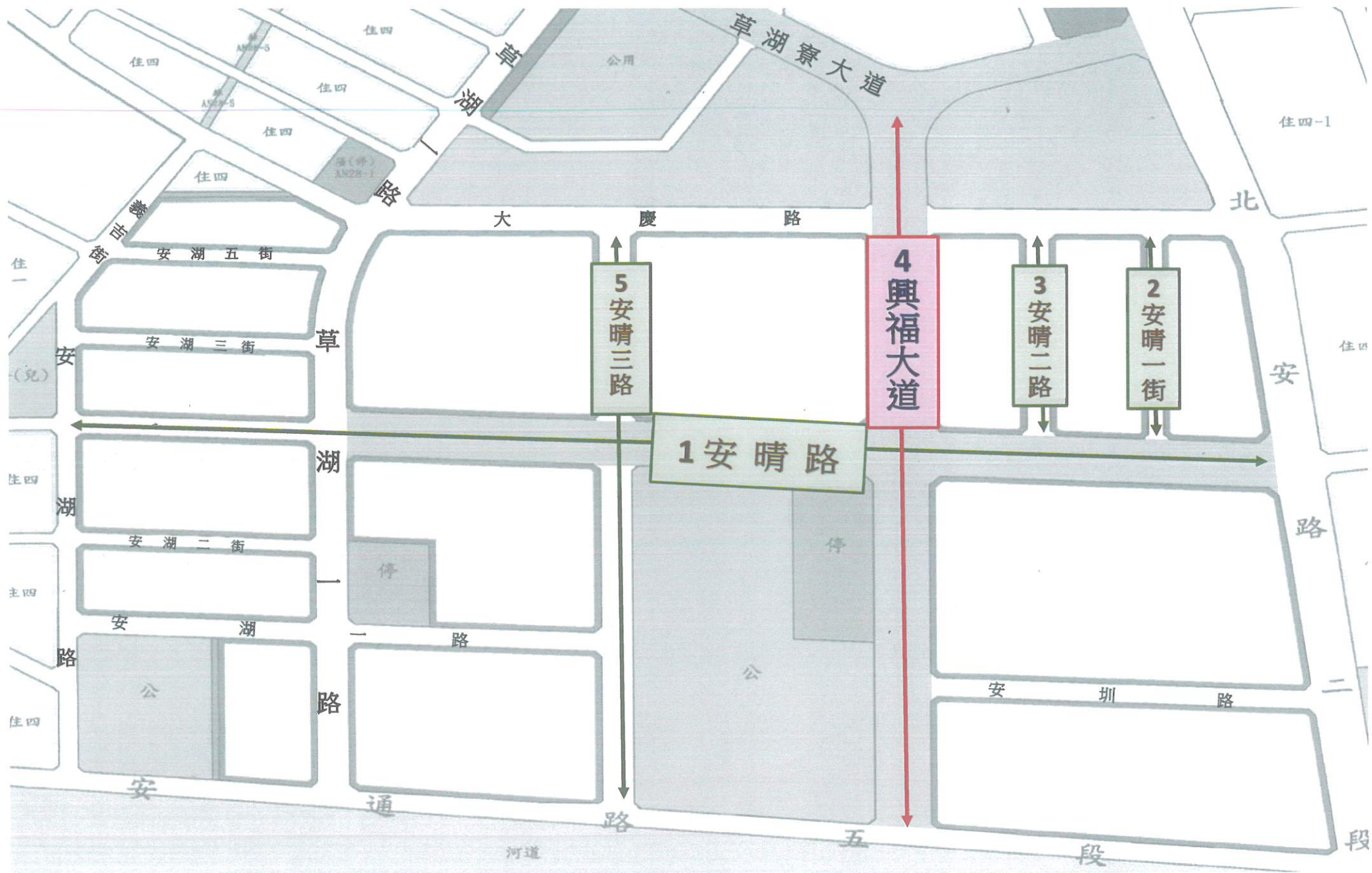
「臺南市第 8 期北安商業區市地重劃區計畫道路」部分道路位置圖
