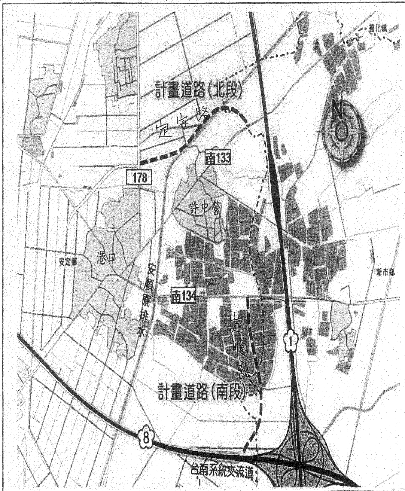
圖 1 南科西向聯絡道路系統示意圖
