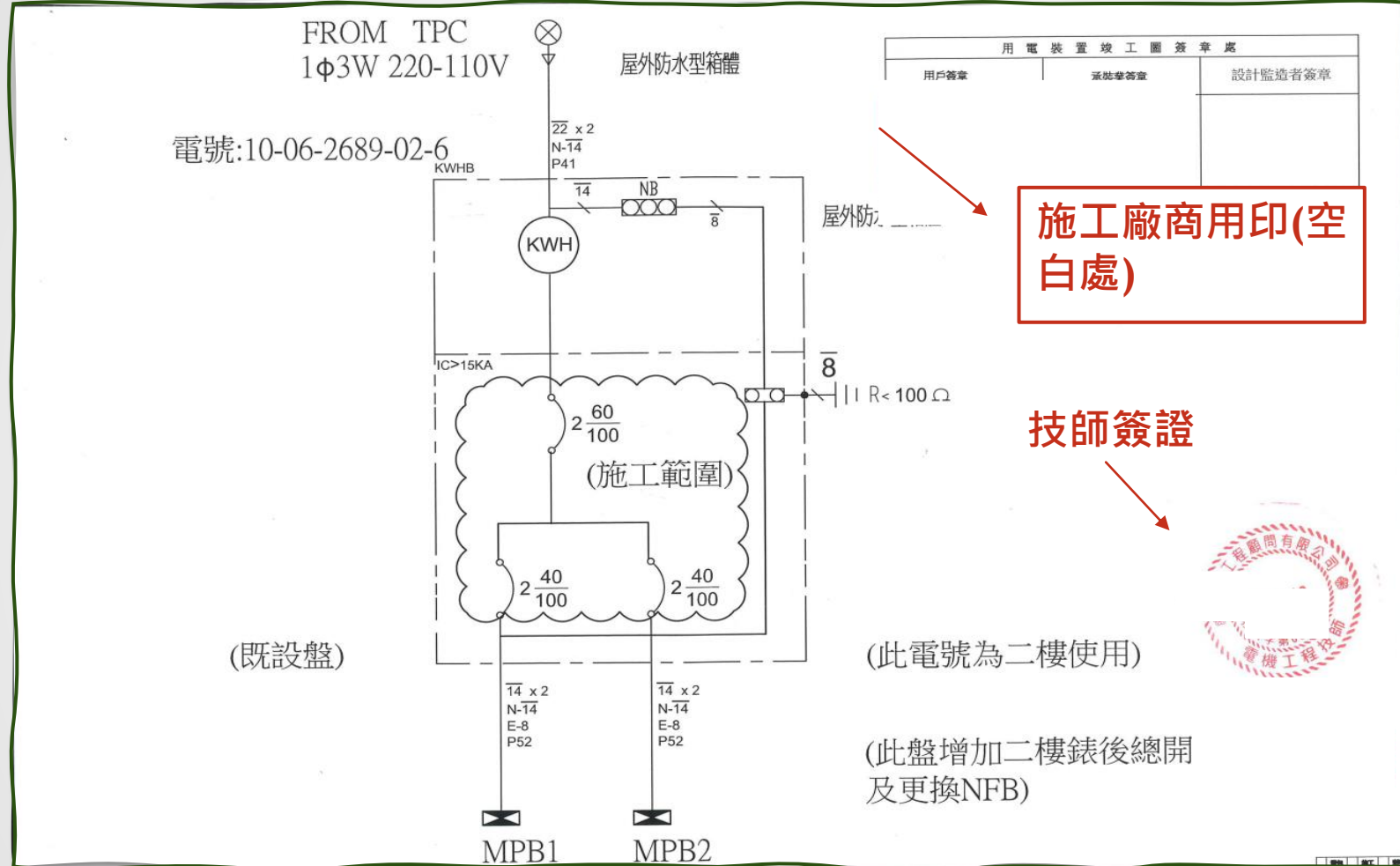
單線圖之竣工圖
