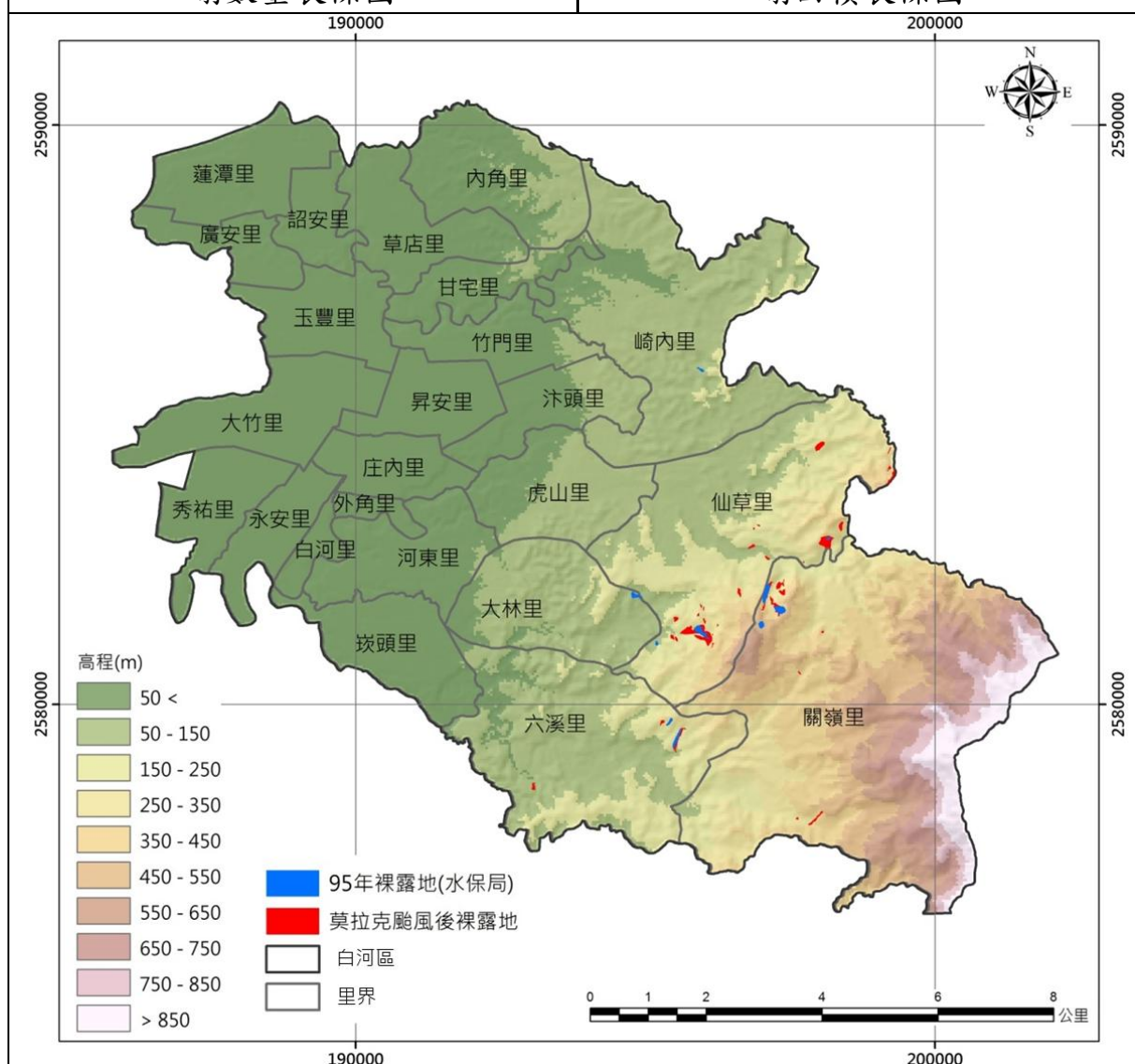
圖 3-1-5、白河區莫拉克颱風前後裸露地位置分佈圖
