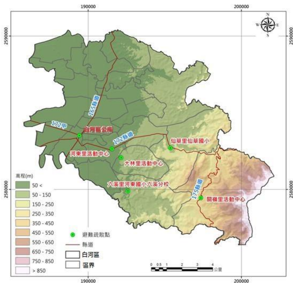
圖 2-1-10、白河區坡地災害避難疏散規劃圖
