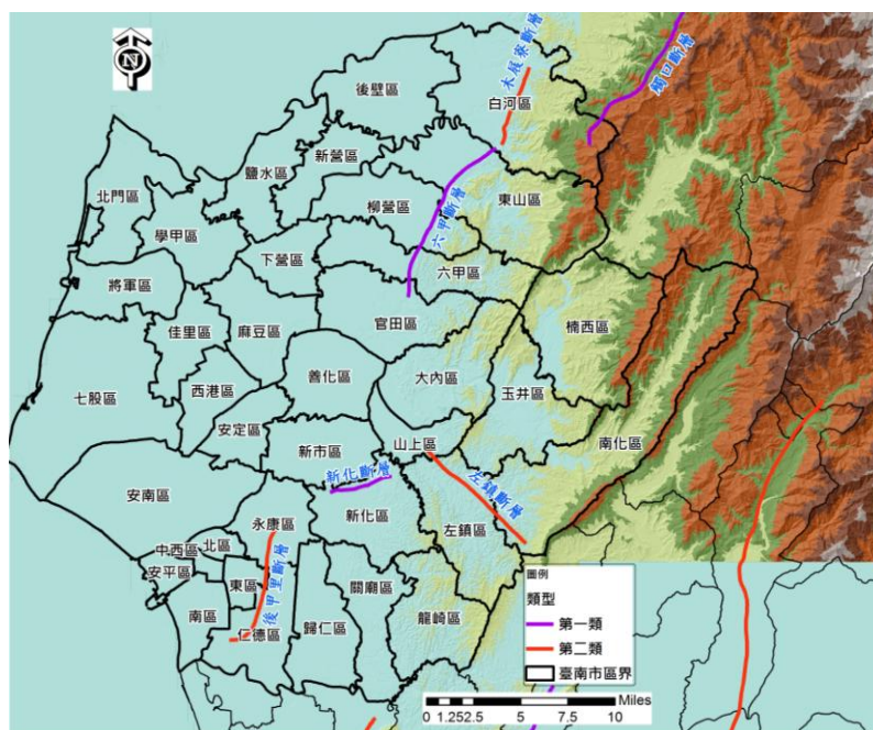
圖 3-6-1、臺南市各地震斷層分佈一覽表
