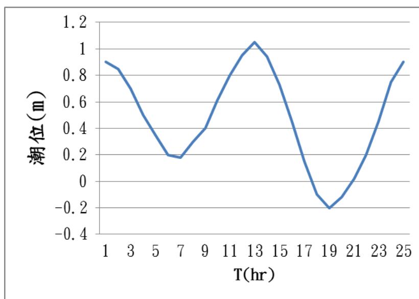
圖 4-1-2、將軍潮位站之平均大潮歷線圖
