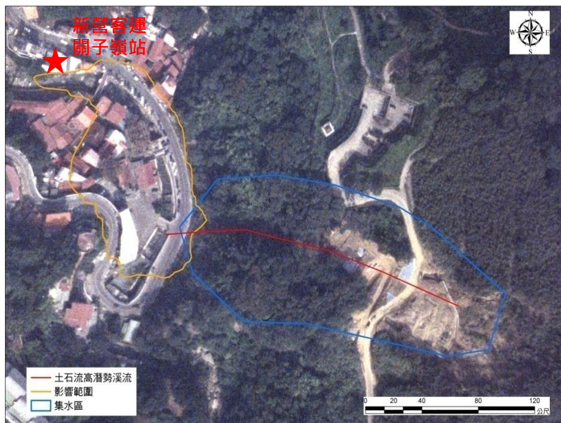
圖 3-6-20、白河區土石流高潛勢溪流南市 DF010 影響範圍圖
