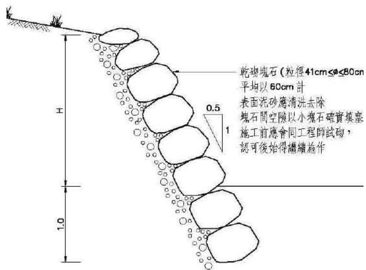
乾砌塊石擋土牆標準圖
