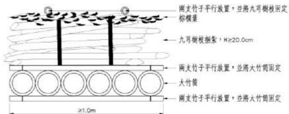
人工魚礁單元示意圖
