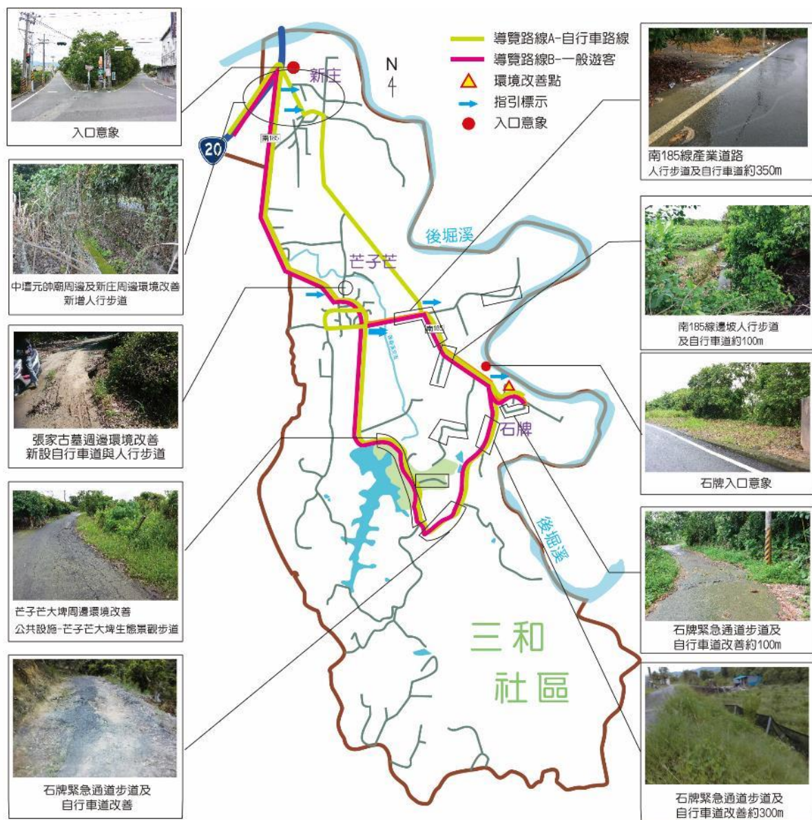
圖 4.4 公共設施建設規劃分布圖
