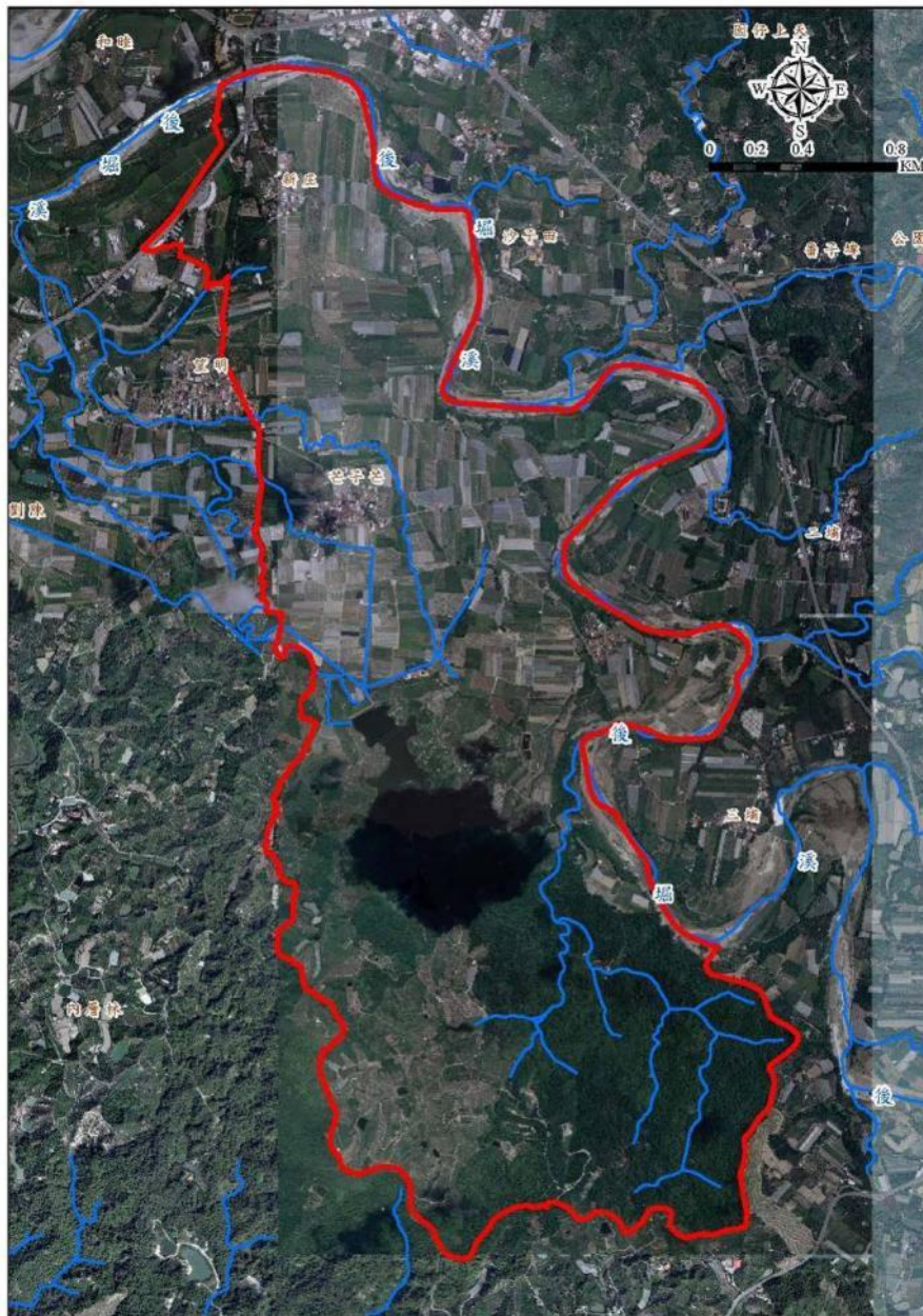
圖 2.9 三和社區水文分布圖
