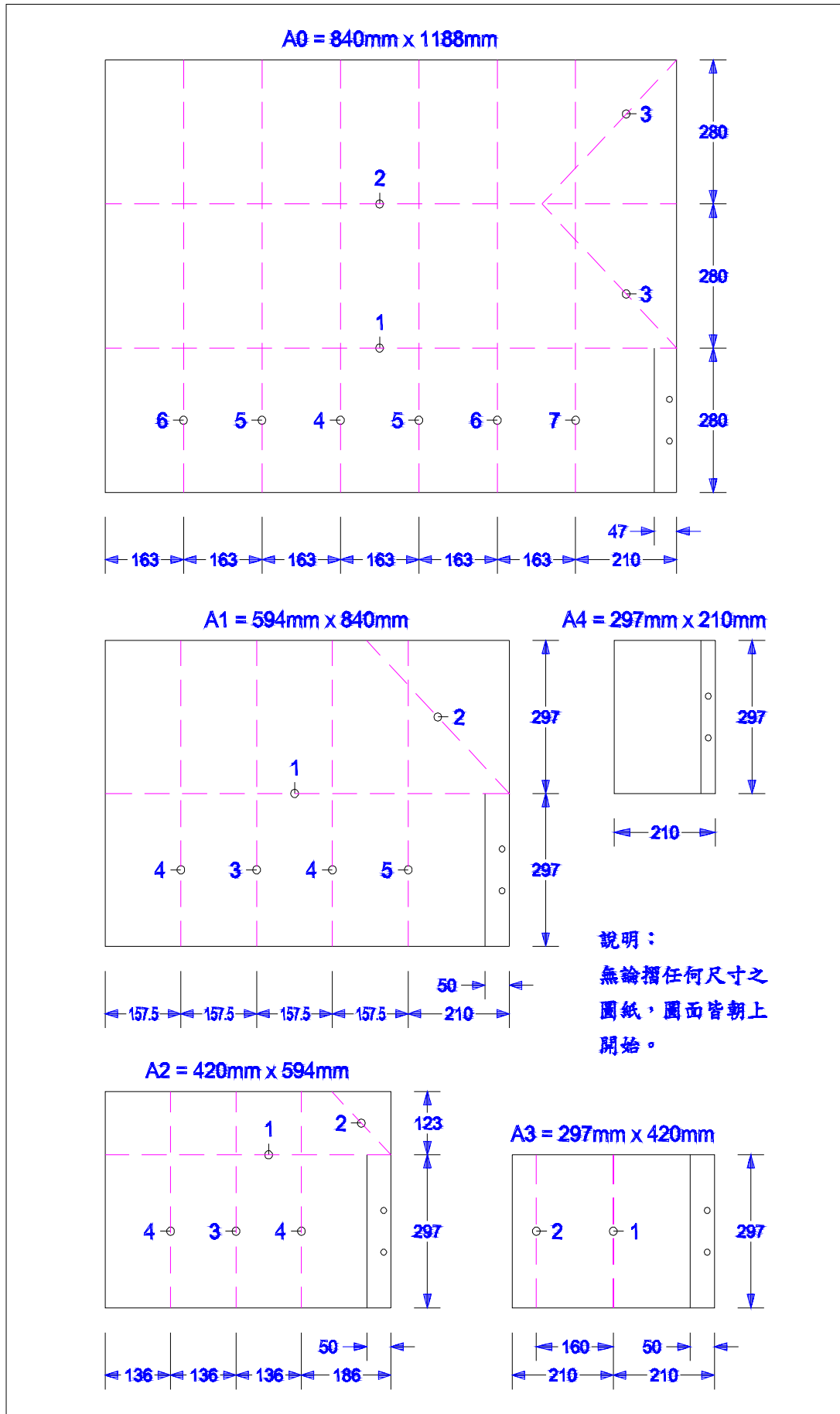
圖三 圖紙摺疊範例
