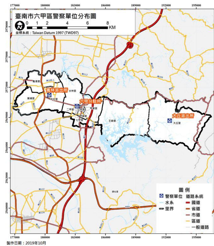
圖 2-1-10、六甲區警察單位分布圖
