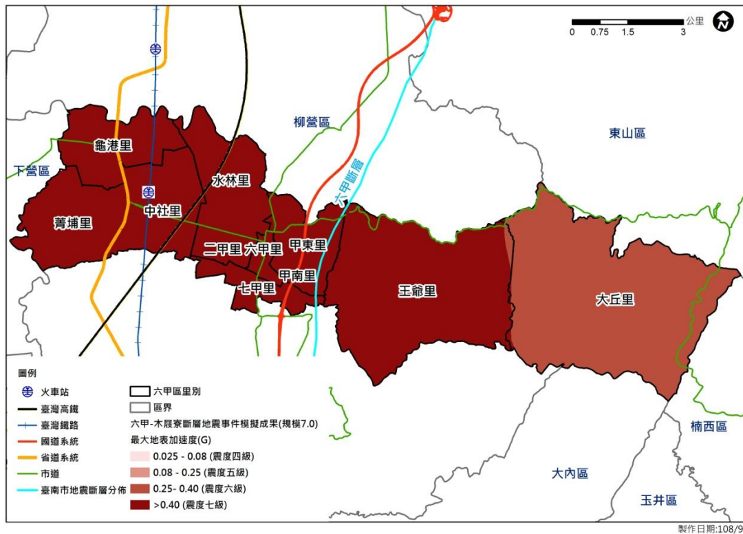
圖 4-1-3、木屐寮-六甲斷層地震事件六甲區最大地表加速度分布圖
