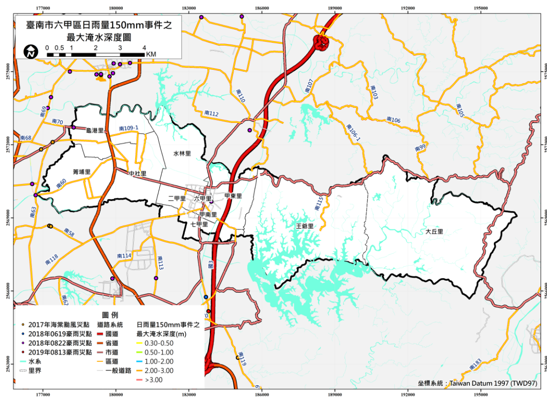
圖 5-1-1、六甲區日雨量 150mm 事件之最大淹水深度圖
