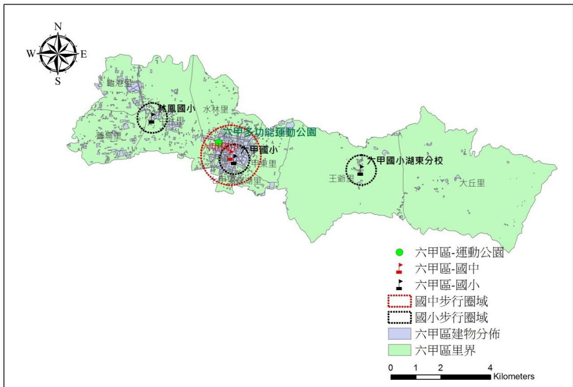
圖 4-1-6、臺南市六甲區可能避難收容地點分佈圖
