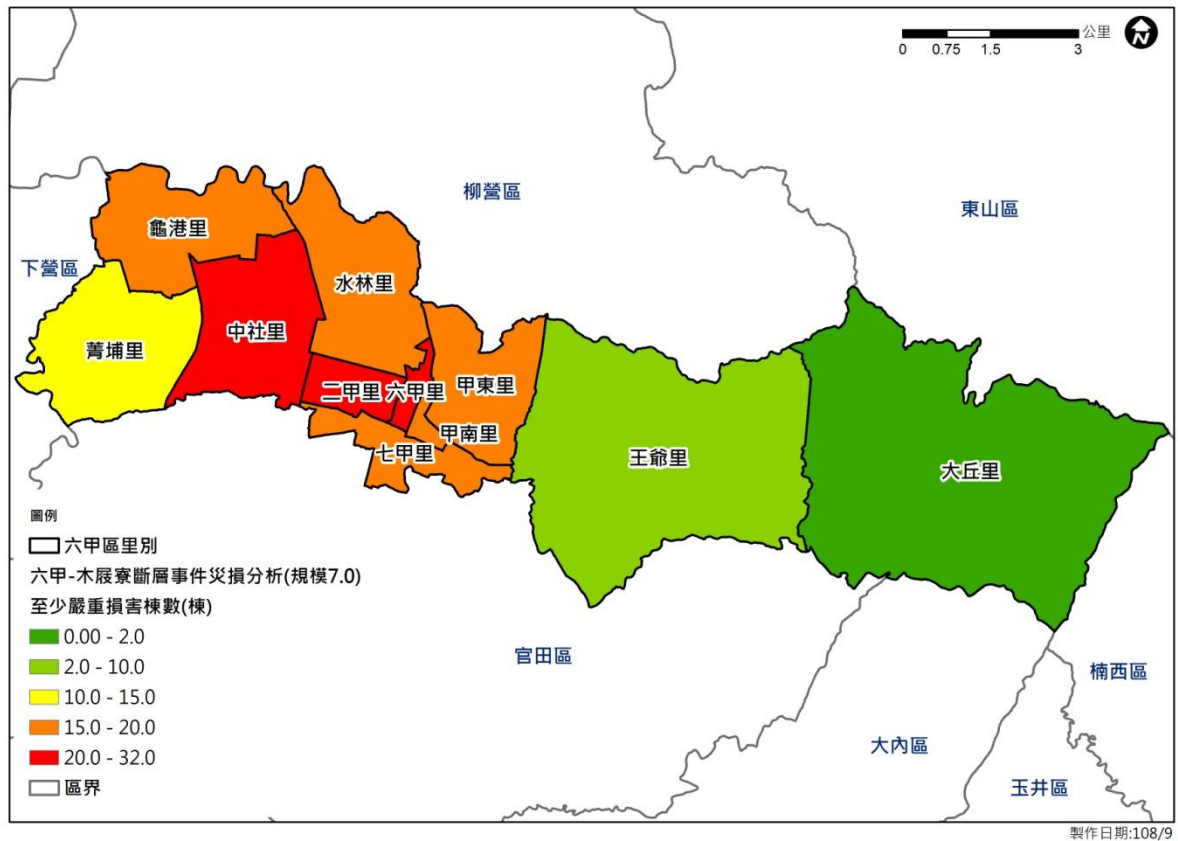
圖 4-1-5、木屐寮-六甲斷層地震建築物至少嚴重損害棟數分布
