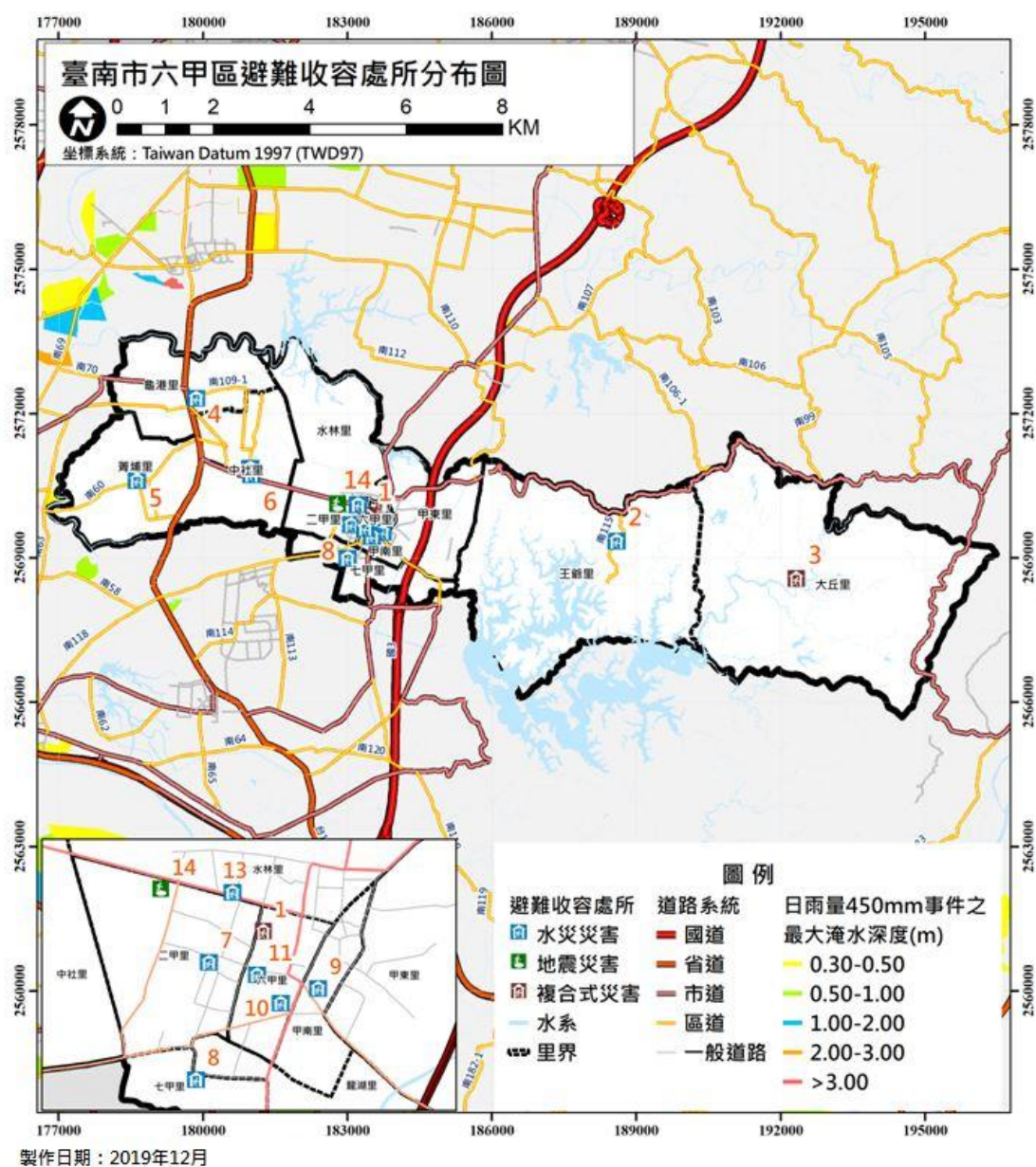
圖 2-1-12、六甲區收容處所分布圖
