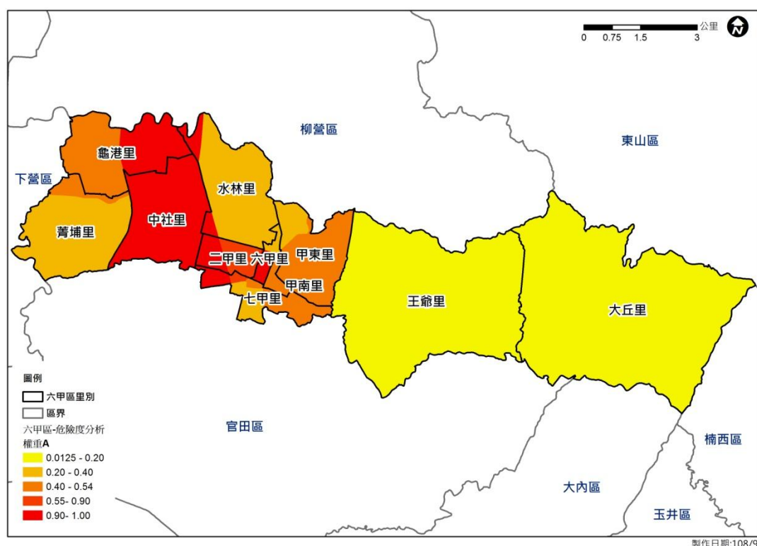
圖 4-1-4、木屐寮-六甲斷層系統地震事件六甲區危險度分布圖
