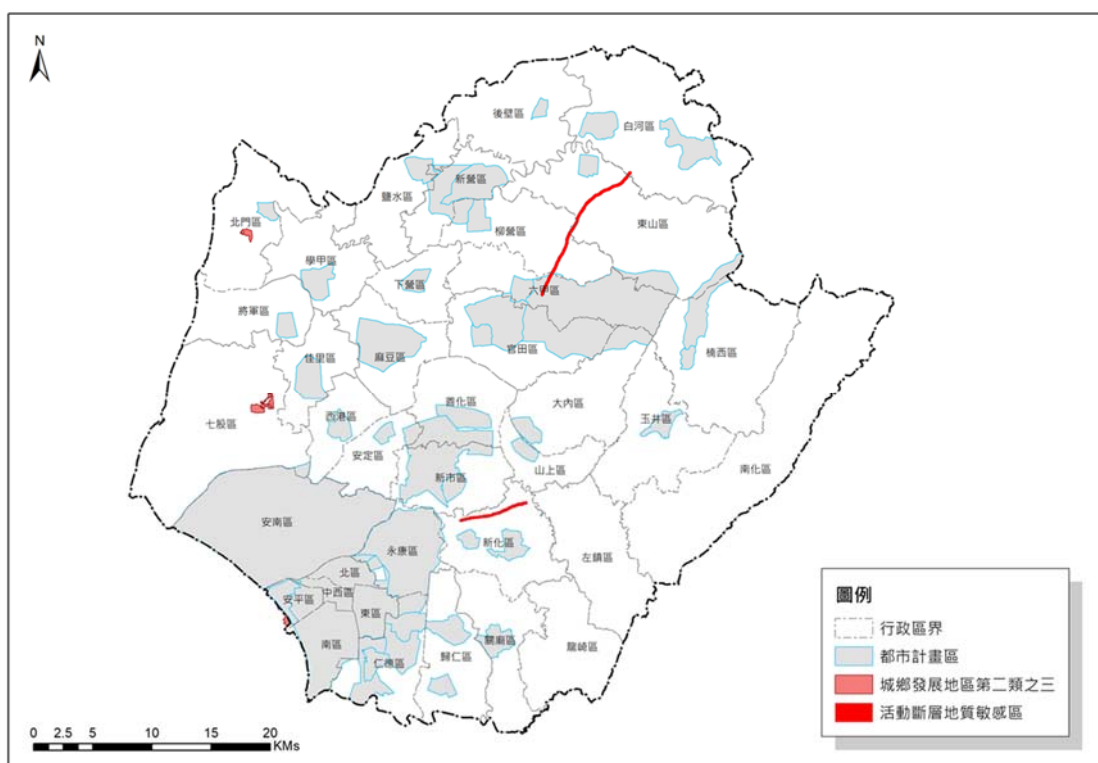
圖 4-6 既有都市計畫區及城鄉發展地區第二類之三(屬新訂或擴大都市計畫範圍)活動斷層地質敏感區分布示意圖
