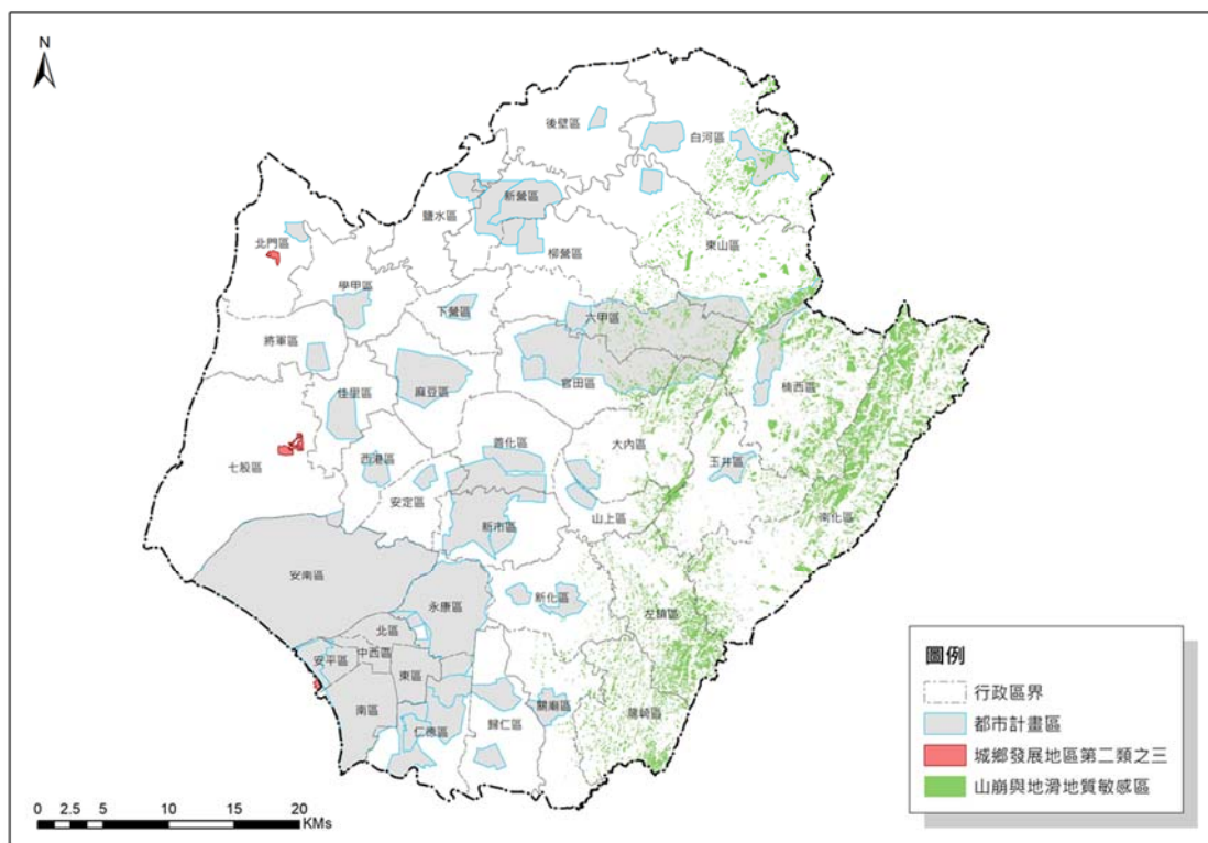
圖 4-5 既有都市計畫區及城鄉發展地區第二類之三(屬新訂或擴大都市計畫範圍)山崩與地滑地質敏感區分布示意圖
