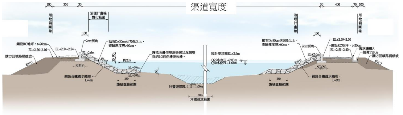
圖 2 劉厝排水 9K+271~10K+555 工程斷面圖
