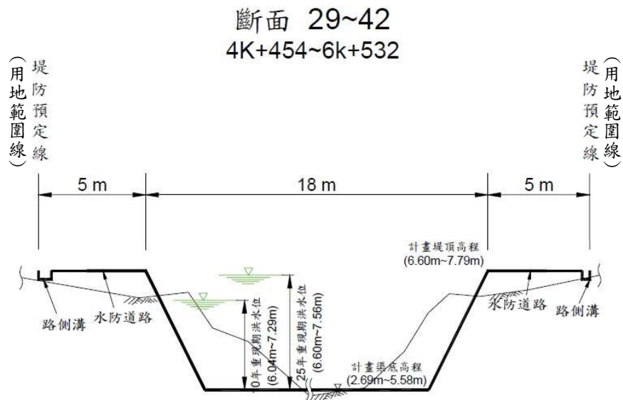
圖 2 本案計畫橫斷圖
