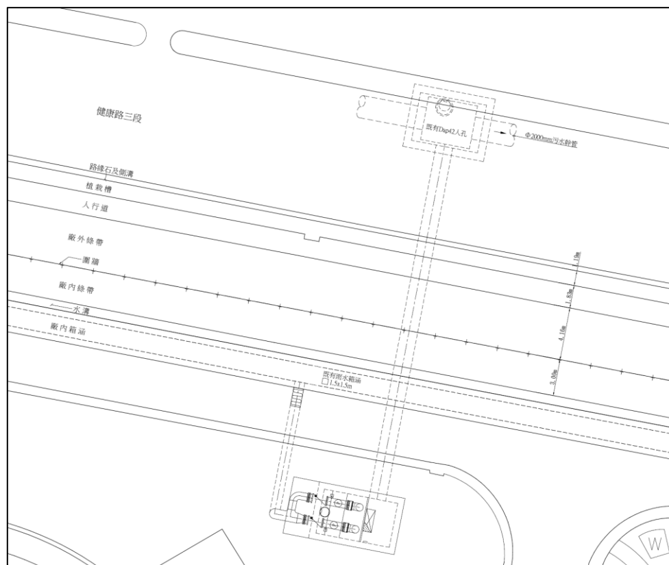
圖 4- 30 安平水資中心疏流規劃設計圖
