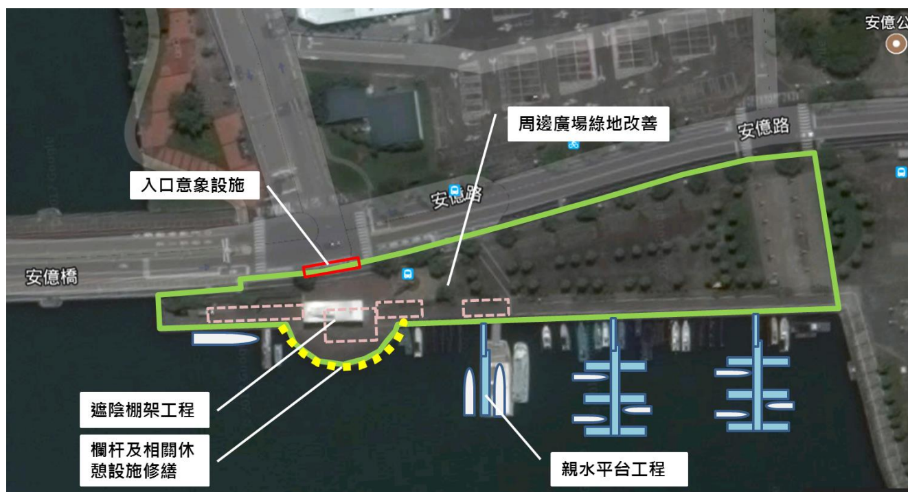
圖 4- 32 安平漁港整體改善構想圖
