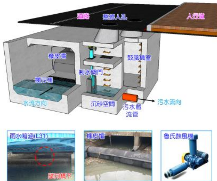
圖 4- 26 雨水箱涵截流
