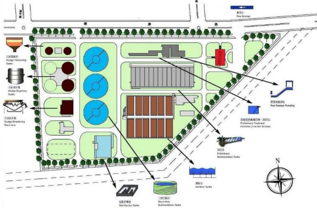
圖 1- 3 安平水資源回收中心配置圖
