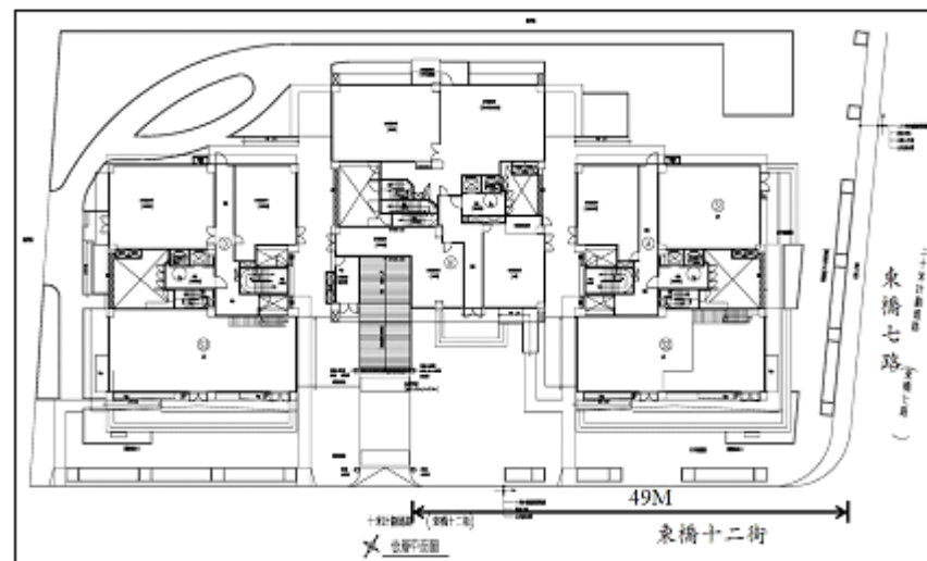
圖4.1.3 基地地下停車場出入口與周邊路口距離示意圖
