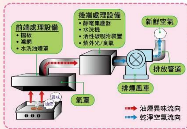
圖 3-1 餐飲業油煙廢氣之處理流程示意圖
