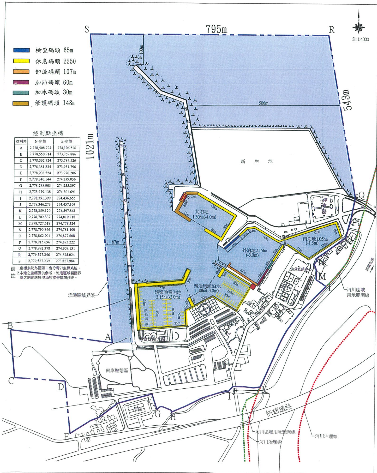
竹圍漁港水域分區使用計畫圖
