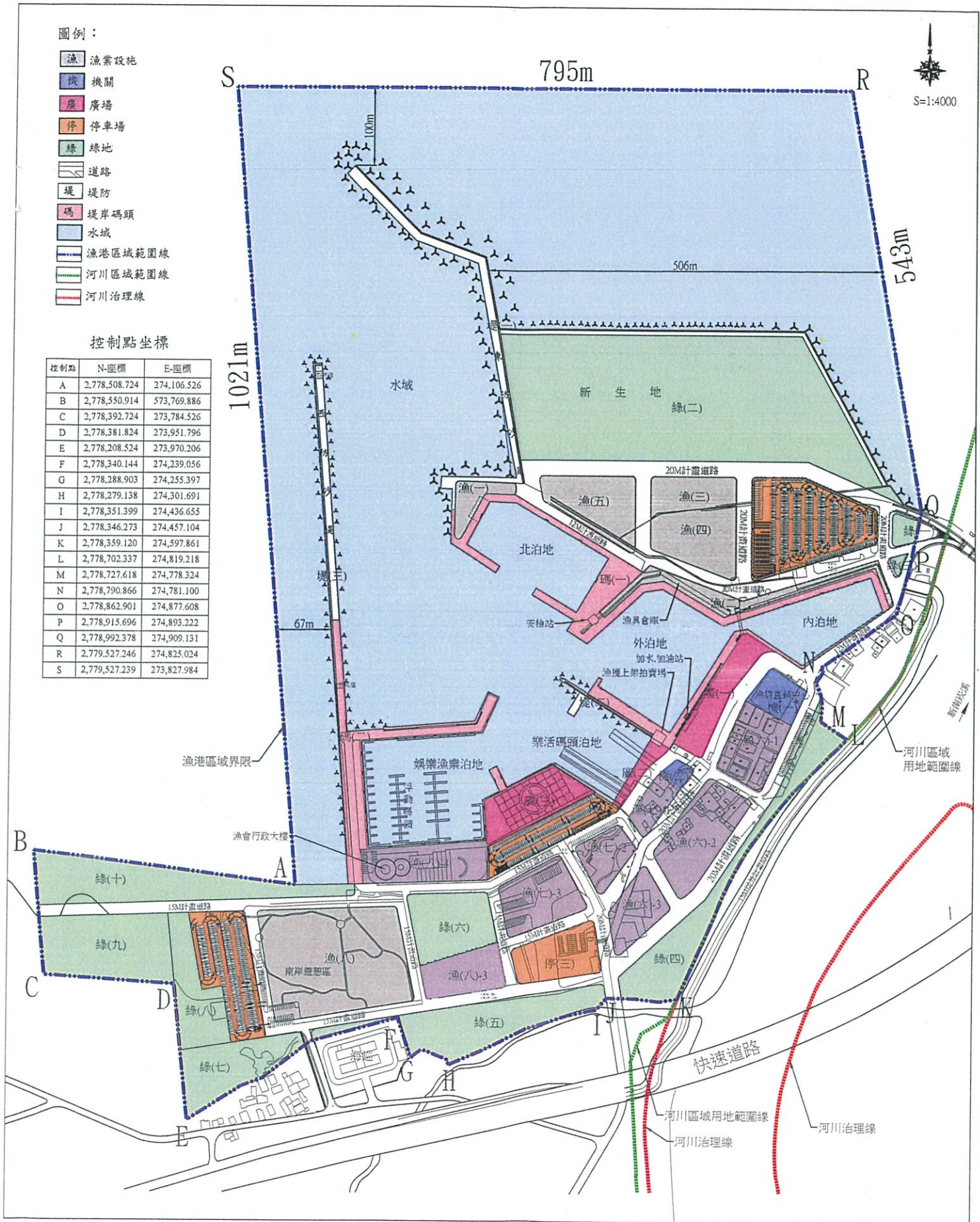
竹園漁港陸域分區使用計畫圖
