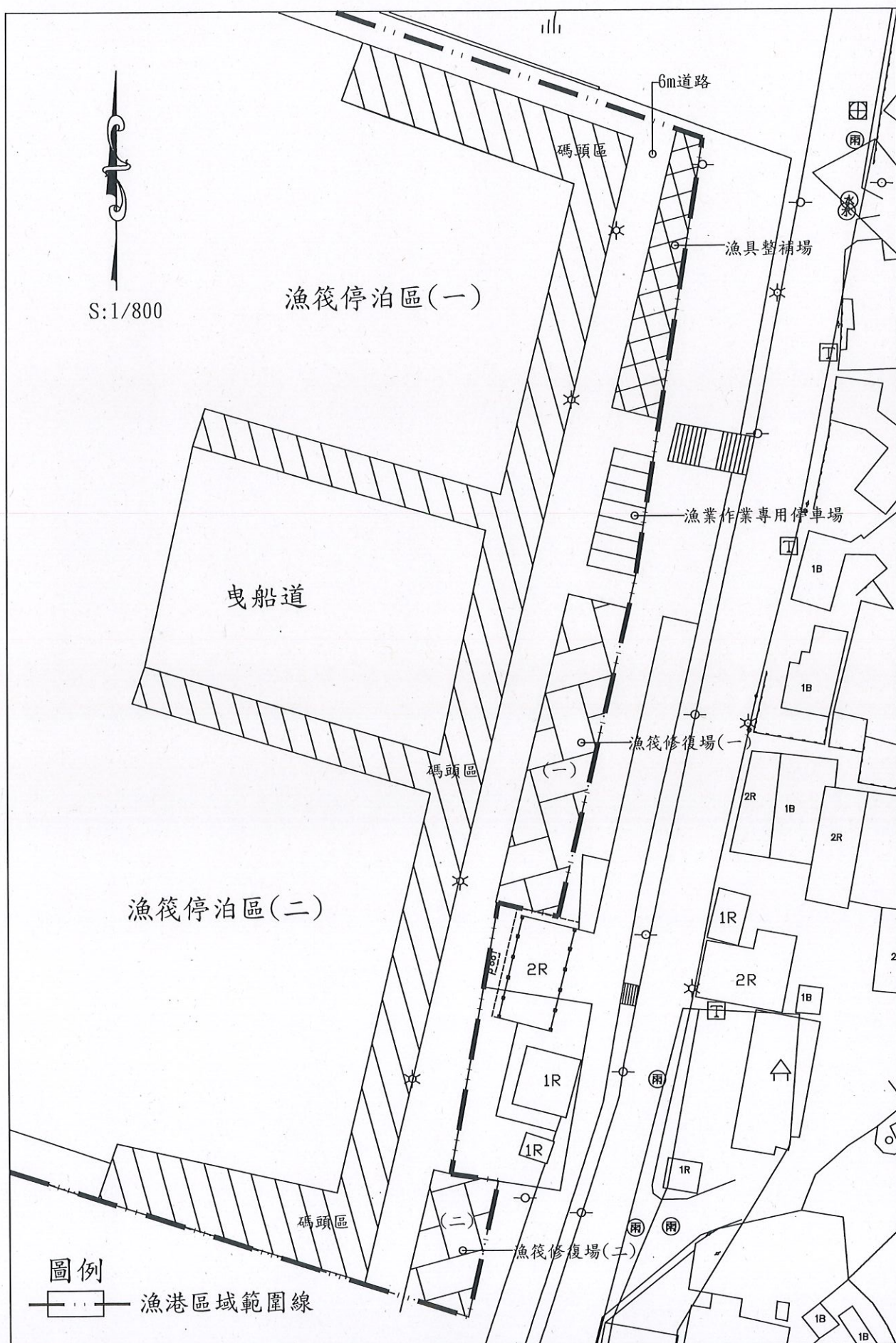
圖七 五甲漁港設施計畫圖
