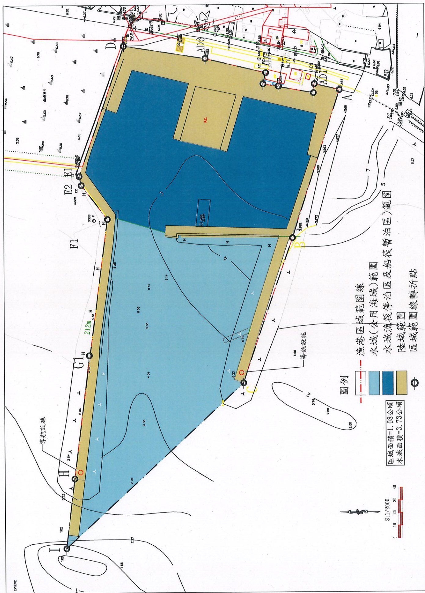
圖三 五甲漁港港區水域及陸域範圍圖
