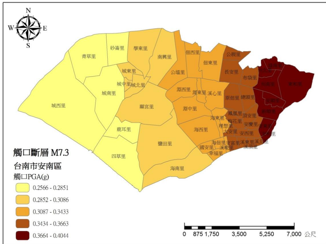
圖 5-1-6、觸口斷層地震事件安南區最大地表加速度分布圖
