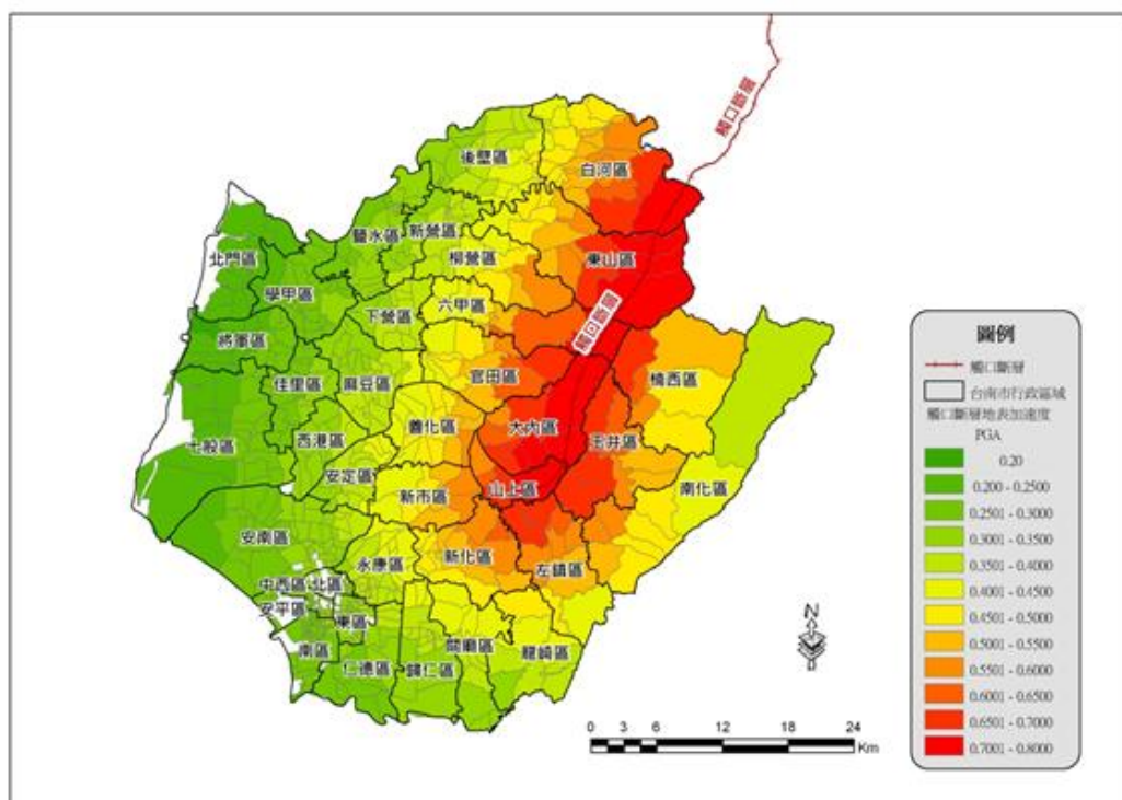
圖 5-1-5、觸口斷層地震最大地表加速度(PGA)分佈圖
