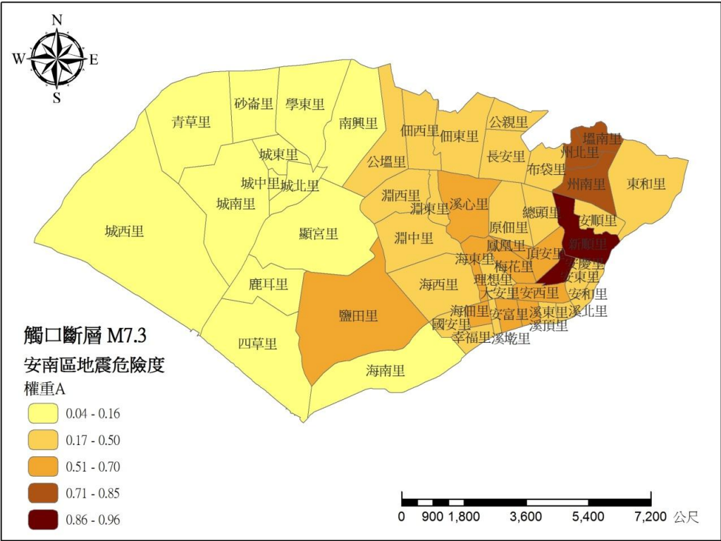
圖 5-1-7、觸口斷層地震事件安南區危險度分布圖
