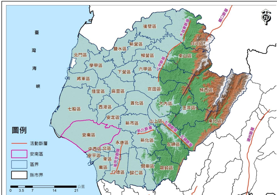
圖 2-1-3、安南區鄰近活動斷層分布圖
