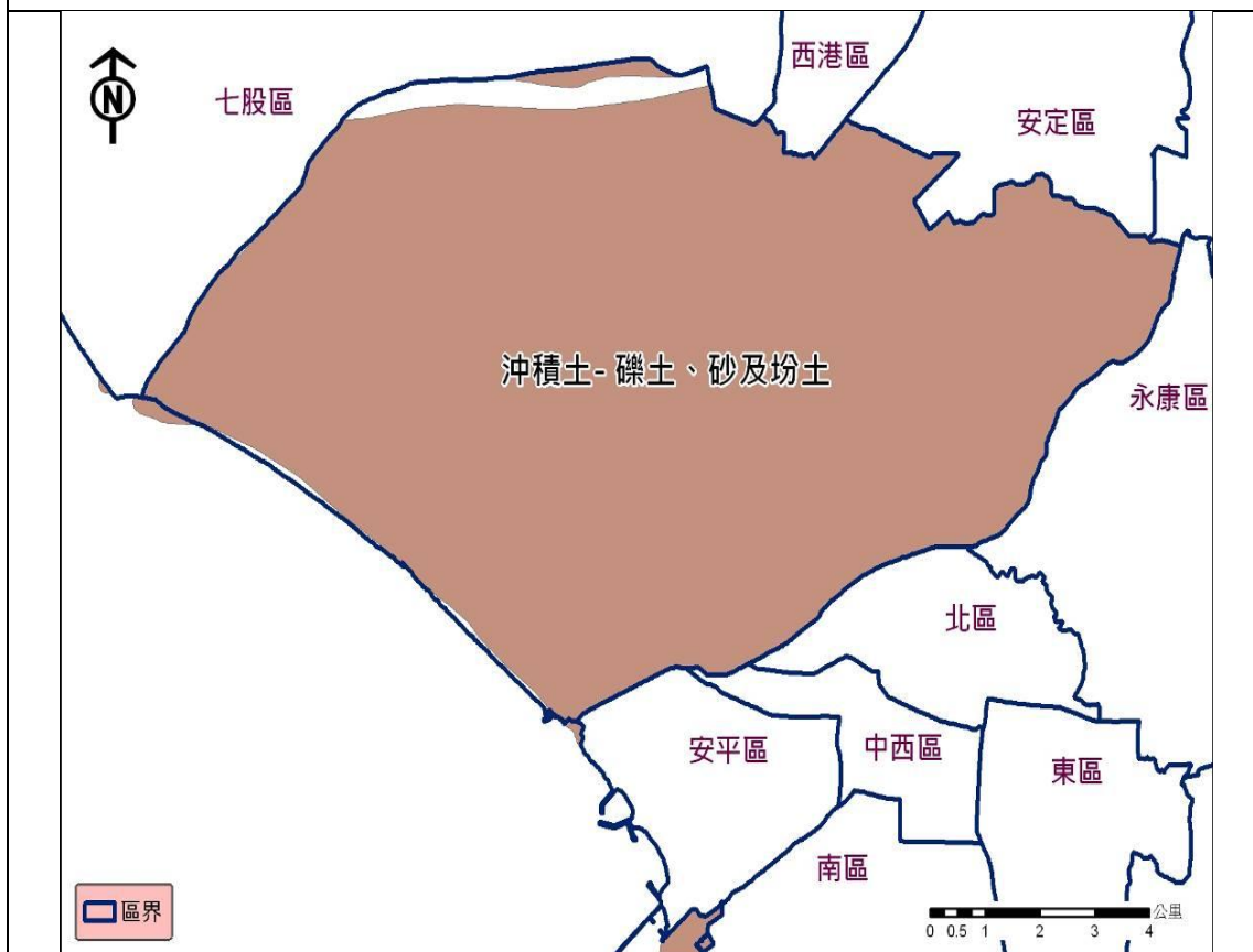
圖 2-1-4、安南區區域地層圖
