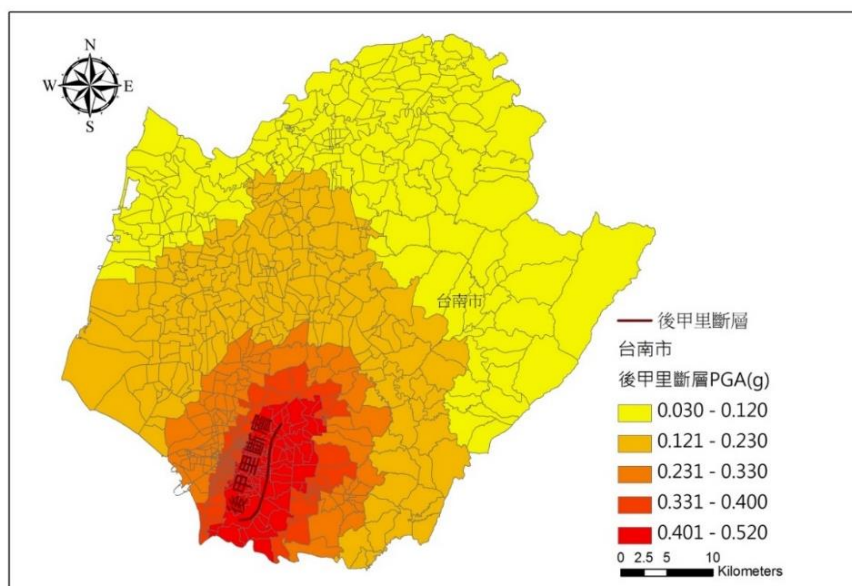
圖 2-2-14 後里斷層地震最大地表加速度(PGA)分佈圖
