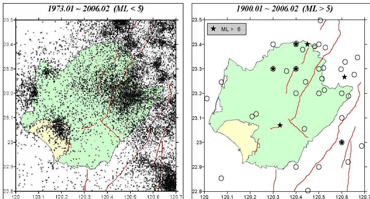
圖 2-2-10 臺南地區的地震活動與斷層分佈
