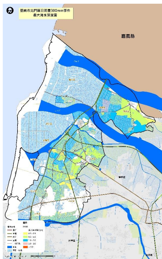
圖 2-2-6 日雨量 300mm 事件之最大淹水深度圖
