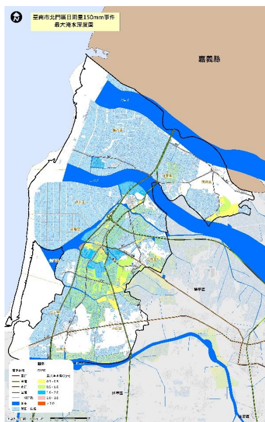
圖 2-2-5 日雨量 150mm 事件之最大淹水深度圖
