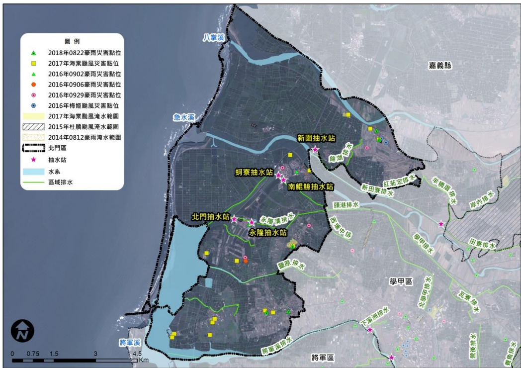
圖 4-5-1 臺南市北門區 2014-2018 年淹水位置圖
