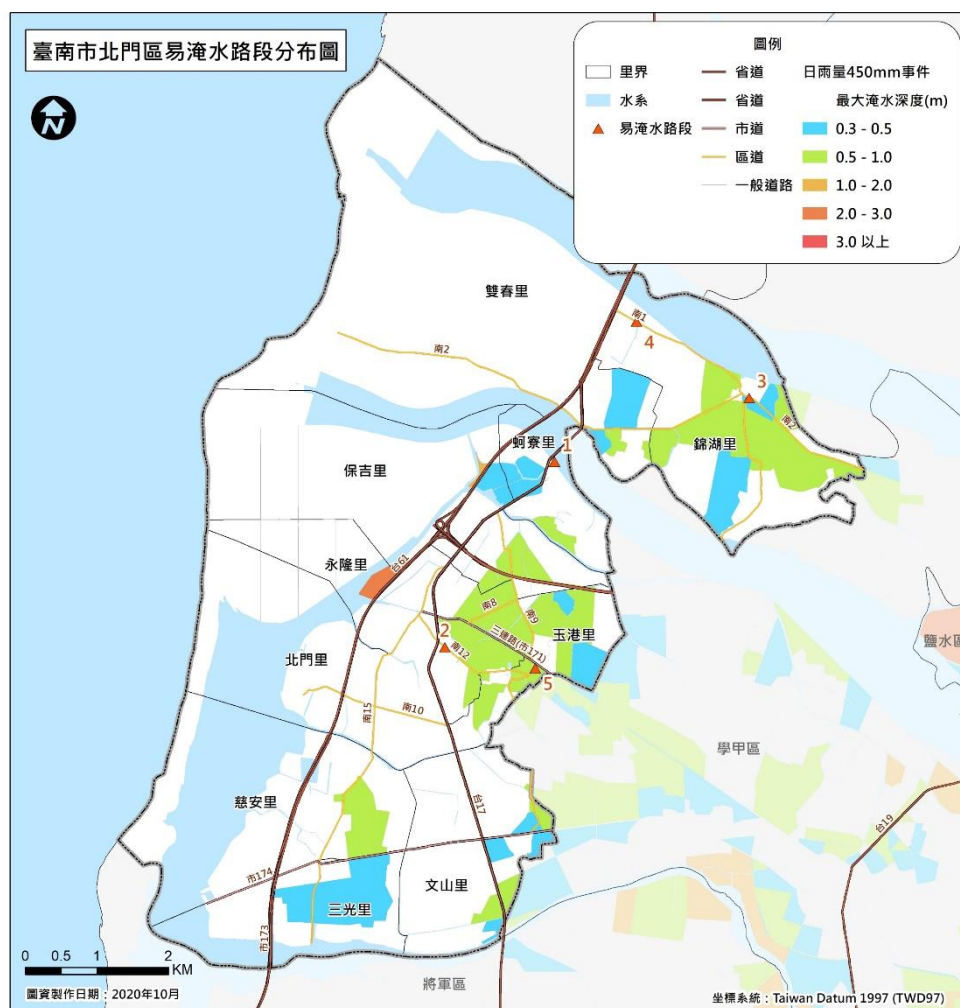
圖 4-1-2 北門區易淹水路段分布圖
