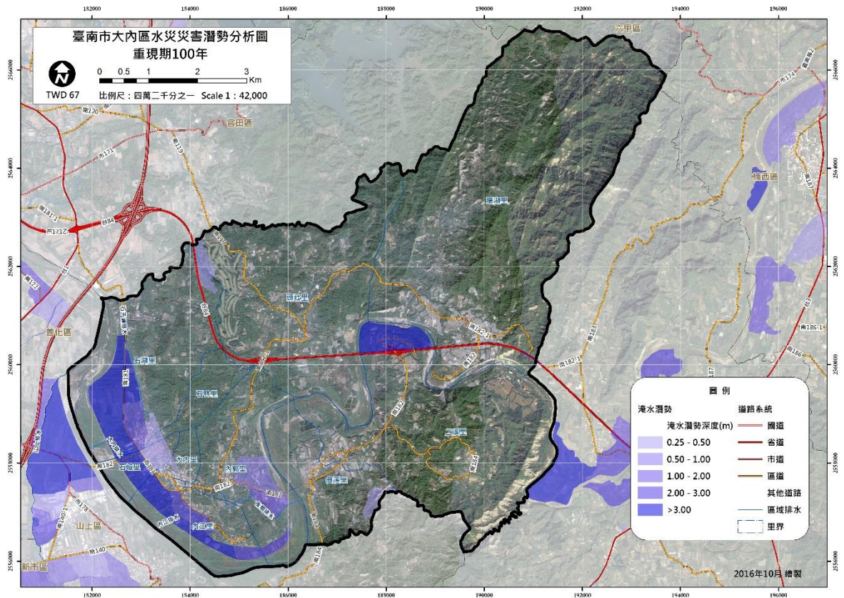
資料來源：臺南市政府 105 年度災害防救深耕計畫 圖 4-1-2 臺南市大內區降雨事件分析圖-重現期 100 年
