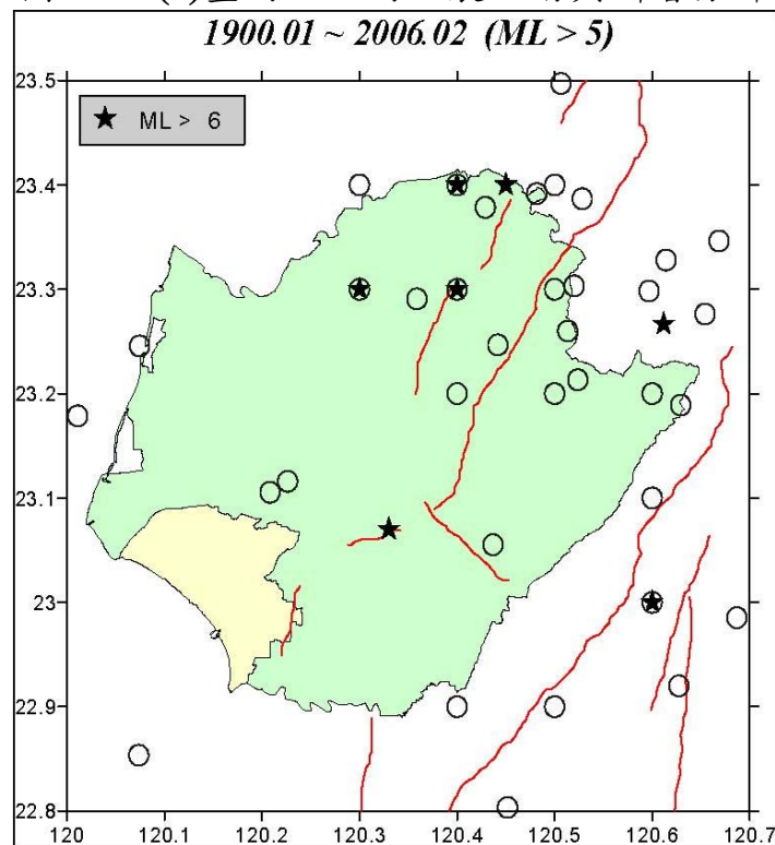
圖 5-1-2(b)臺南地區的地震活動與斷層分佈
