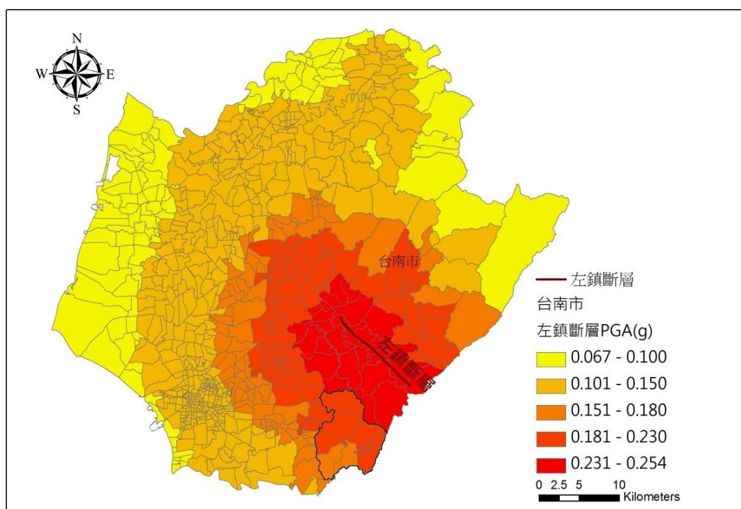
圖 5-1-3 左鎮斷層地震最大地表加速度(PGA)分佈圖
