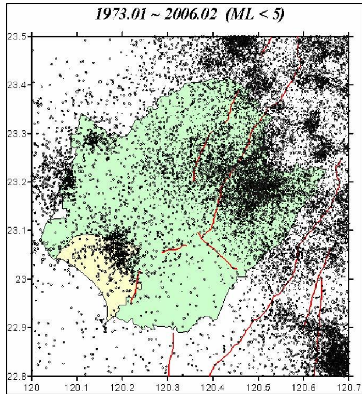
圖 5-1-2(a)臺南地區的地震活動與斷層分佈
